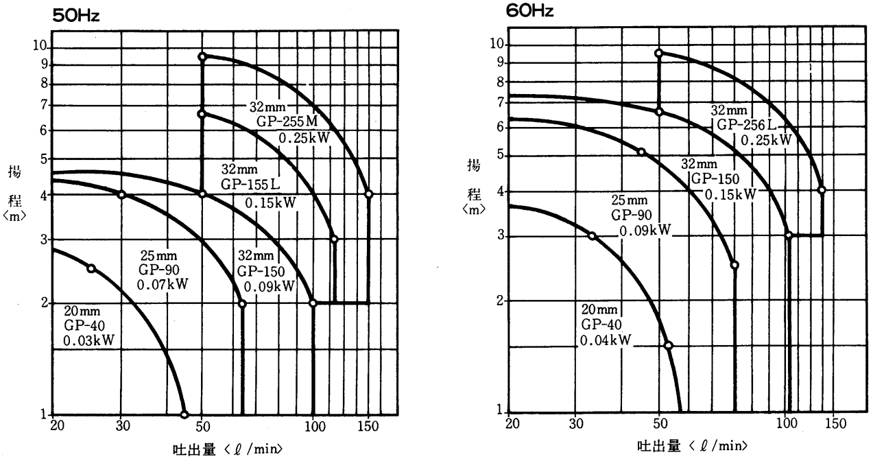
図4 GP形循環ポンプ選定図
