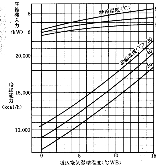
GT-100C形冷却能力線図<風量210m 3 /min> 50Hz
