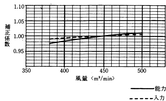
風量補正線図
