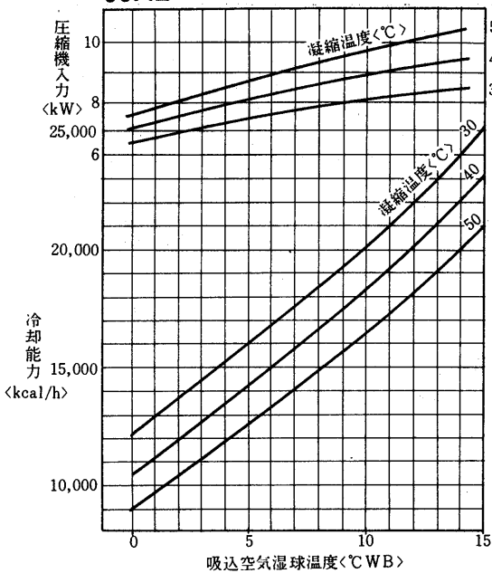
冷却能力線図<風量210m 3 /min> 60Hz
