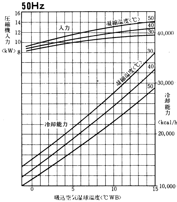
GT-150C形冷却能力線図
