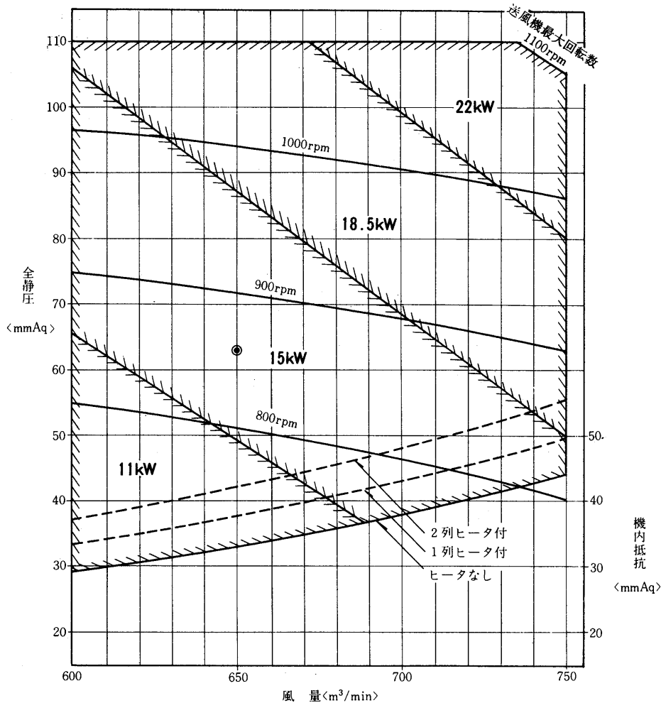
送風機性能線図
