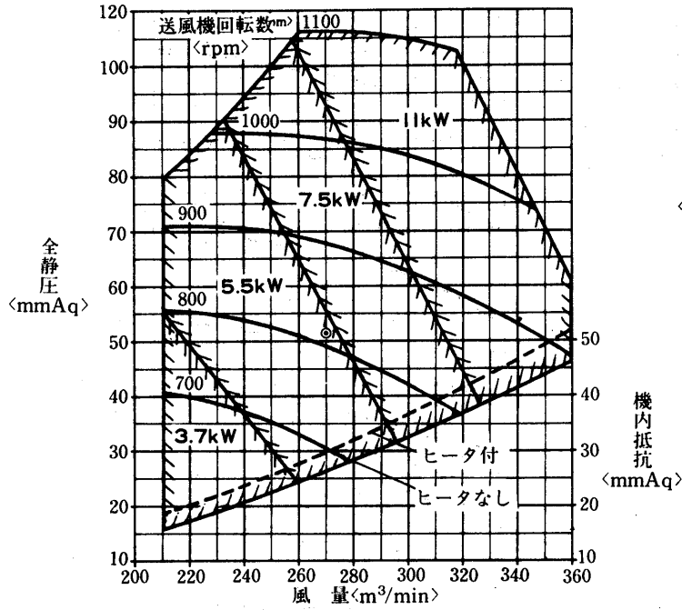
送風機性能線図
