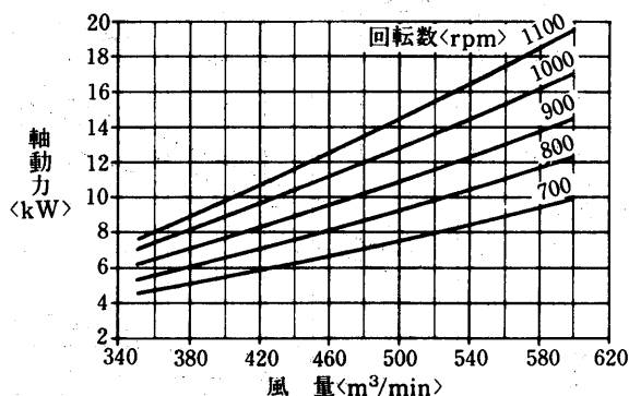
送風機軸動力線図
