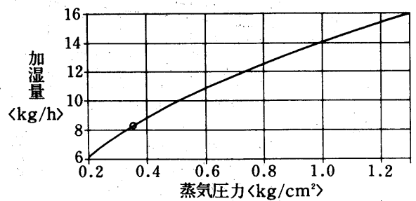
蒸気加湿器能力線図<別売部品>
