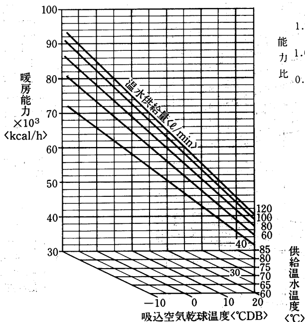
温水加熱器能力線図<別売部品>
