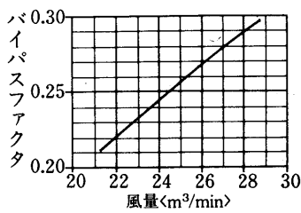
バイパスファクタ線図 <50/60Hz>
