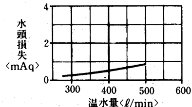
水頭損失線図
