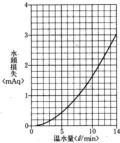
水頭損失線図
