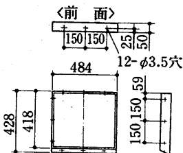
後吸込ダクトフランジ
