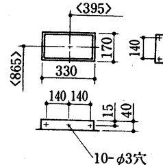
ダクトフランジ<外気取入> <別売部品>
