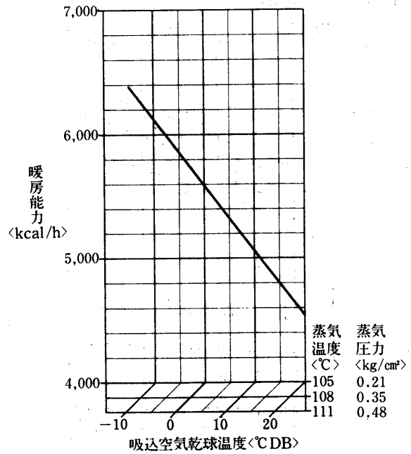
蒸気加熱器能力線図<別売部品>
