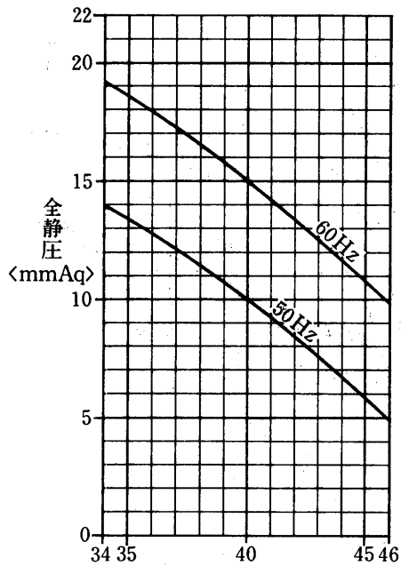
送風機性能線図
