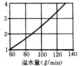
水頭損失線図
