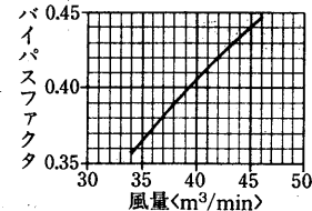
バイパスファクタ線図 <50/60Hz>
