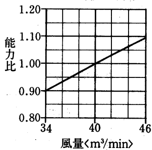
風量補正線図
