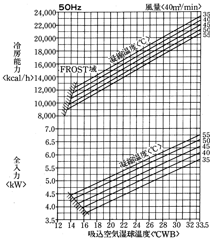
MB-150TA形冷房能力線図
