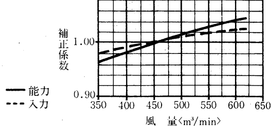
風量補正線図
