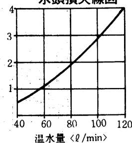
水頭損失線図
