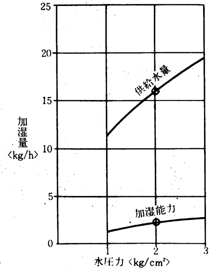
温水加湿器能力線図<別売部品>
