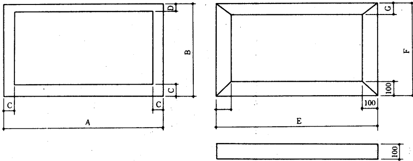
変化寸法表
