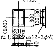
外気取入フランジ <別売部品> <135>
