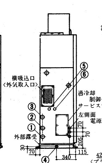
外気取入フランジ <別売部品> <135>
