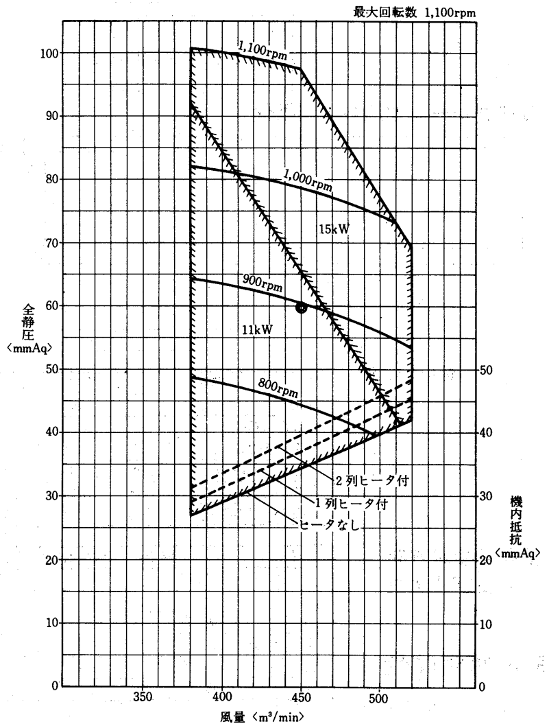
送風機性能線図
