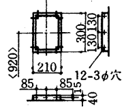
外気取入フランジ <別売部品> <135>
