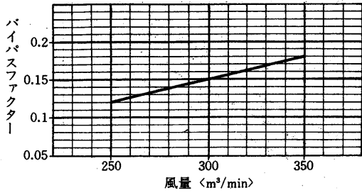
バイパスファクタ線図<50・60Hz>
