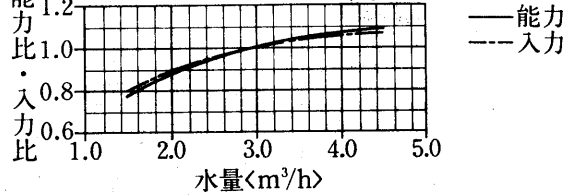
水量補正線図
