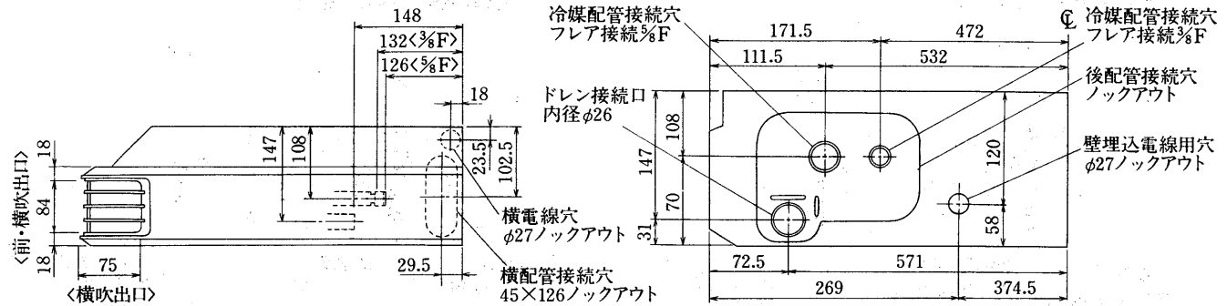
変化寸法表
