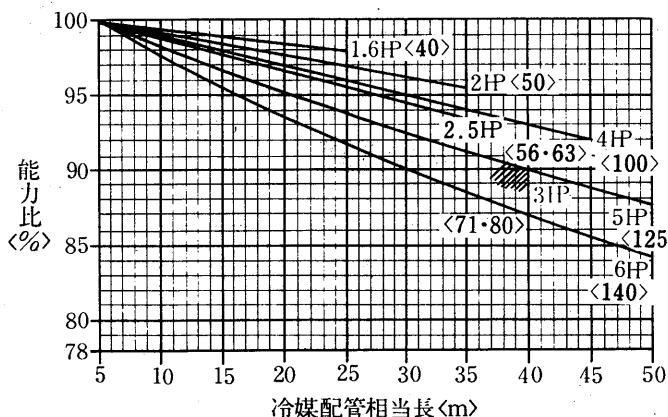
冷房時 50Hz
