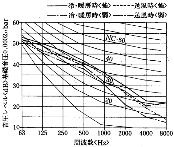
PWH-3B形
