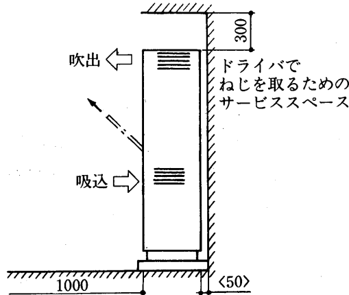
エアフィルタ着脱 本体サービススペース
