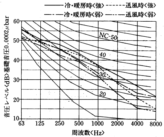
PWH-5A 2 形
