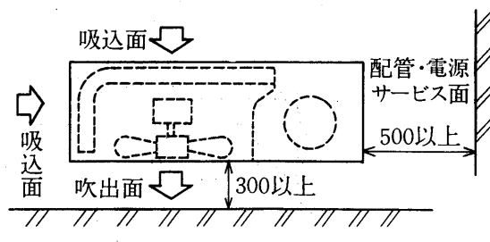
吹出面を壁側に据付けた場合
