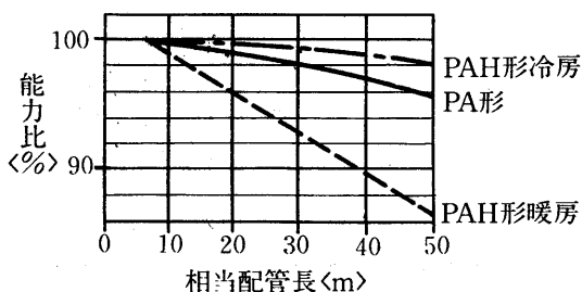
PA<H>-5形
