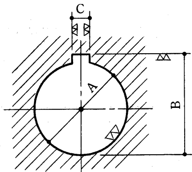
(e)送風機側プーリ ポス部形状
