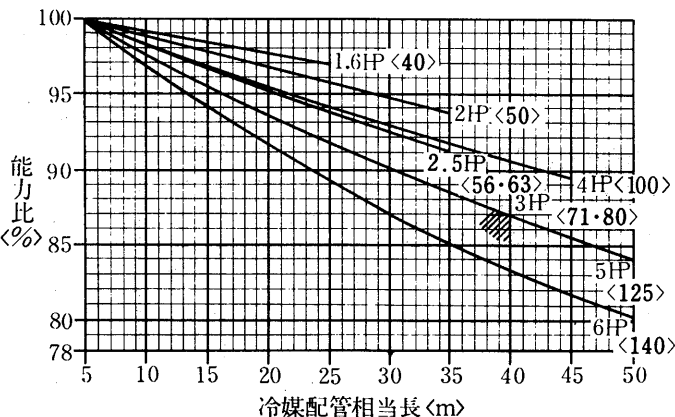
冷房時 60Hz
