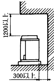
(ロ) 上面〈吹出側〉および側面〈吸込側〉の一方に障害物あり
