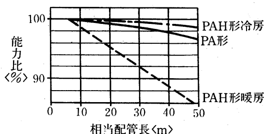
PA<H>-8・15形
