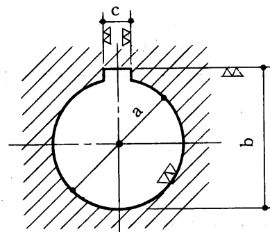
(e)送風機側プーリ ポス部形状
