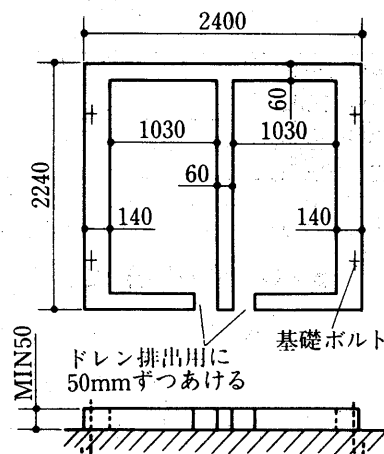
基礎図<PAH-40E・50E形>
