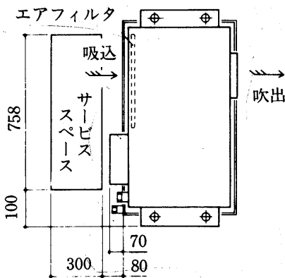
MB形
