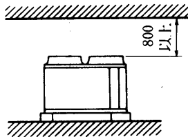
(イ) 上面〈吹出側〉のみ障害物あり
