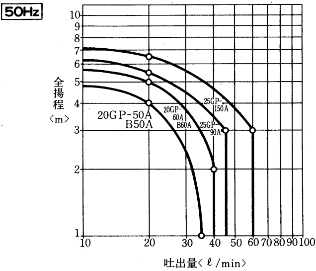
図 4 LPS形循環ポンプ選定図
