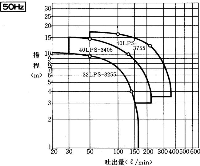
図 5 CP形自吸式うず流れポンプ選定図
