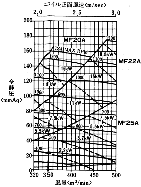
AD-450MA-V形 〈シロツコ1連ファン〉
