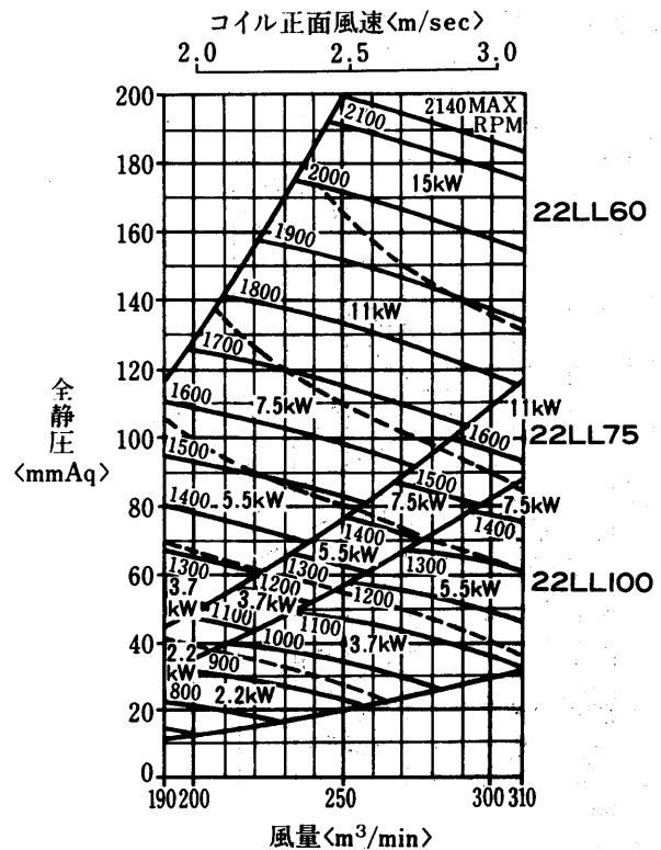
AD-270MA-H形 <リミットロード(LL)ファン>
