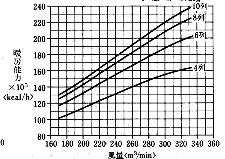
温水コイル選定図 <温水60°C>
