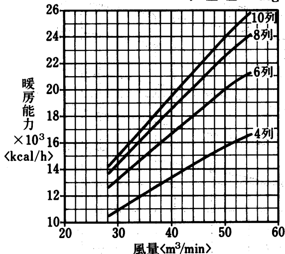
温水コイル選定図 <温水45°C>
