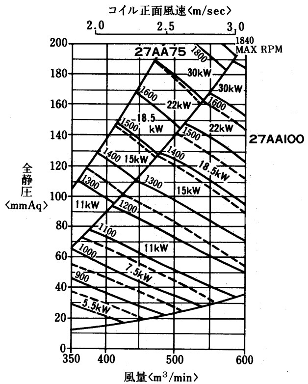
AD-530MA-V形 〈エアホイル(AA)ファン〉
