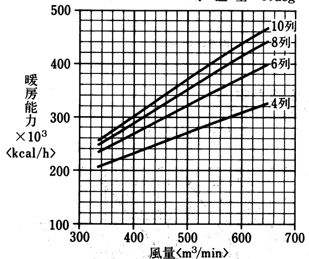
温水コイル選定図 <温水60°C>
