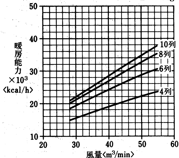
温水コイル選定図 <温水60°C>
