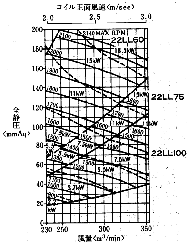
AD-300MA-H形 <リミットロード(LL)ファン>
