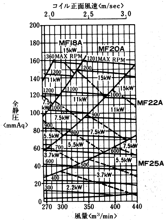
AD-380MA-H形 <シロッコ1連ファン>
