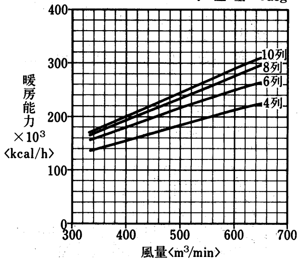
温水コイル選定図 <温水45°C>
