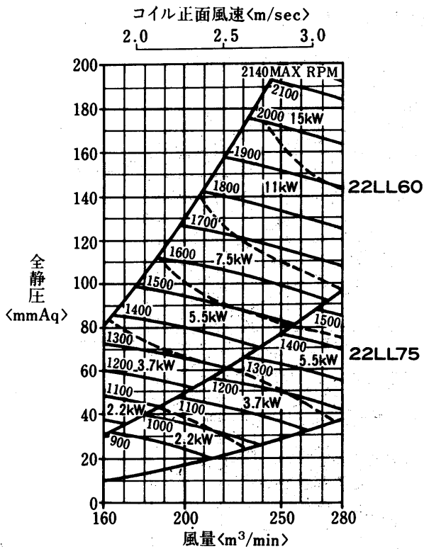
AD-240MA-H形 <リミットロード(LL)ファン>
