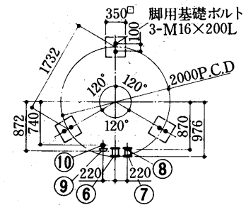
基礎希望図
