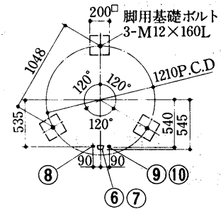
基礎希望図
