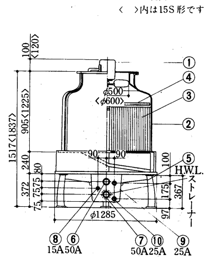
基礎希望図
