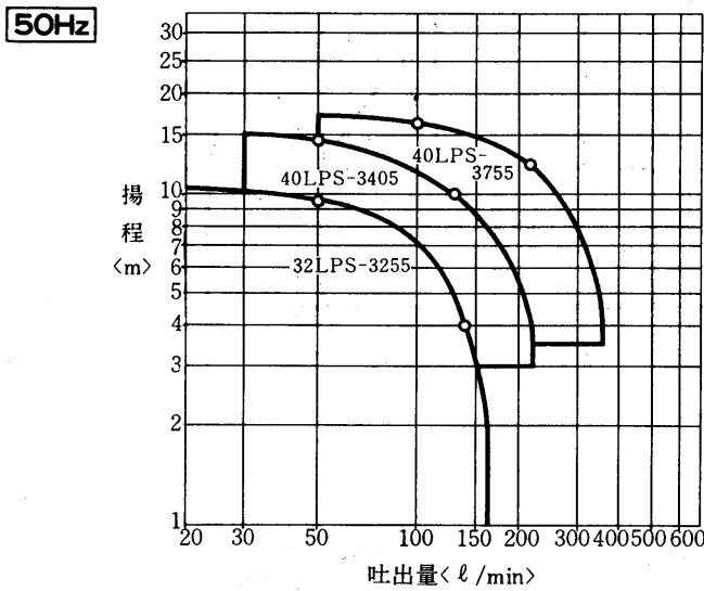
図 5 CP形自吸式うず流れポンプ選定図
