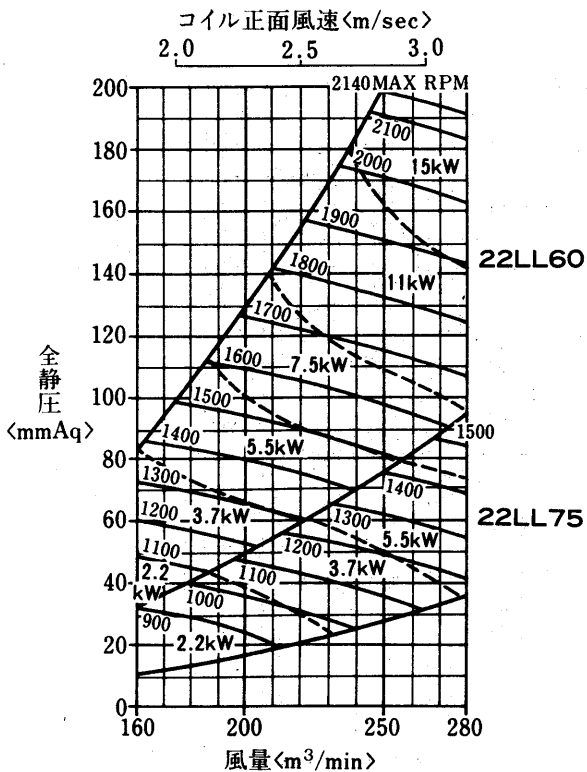
AD-240MA-V形 〈リミットロード(LL)ファン〉
