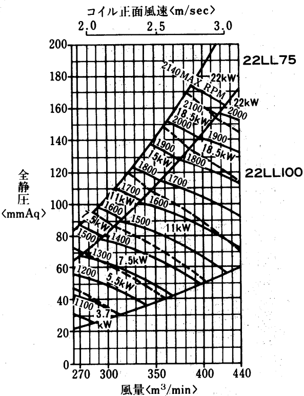
AD-380MA-V形 〈リミットロード(LL)ファン〉
