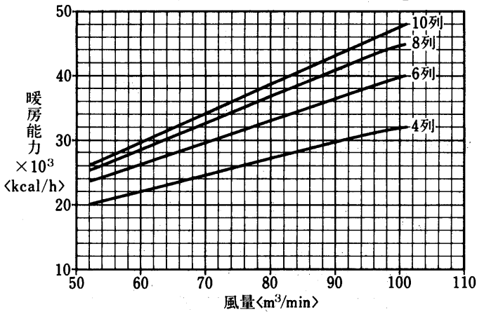
温水コイル選定図 (温水45°C)
