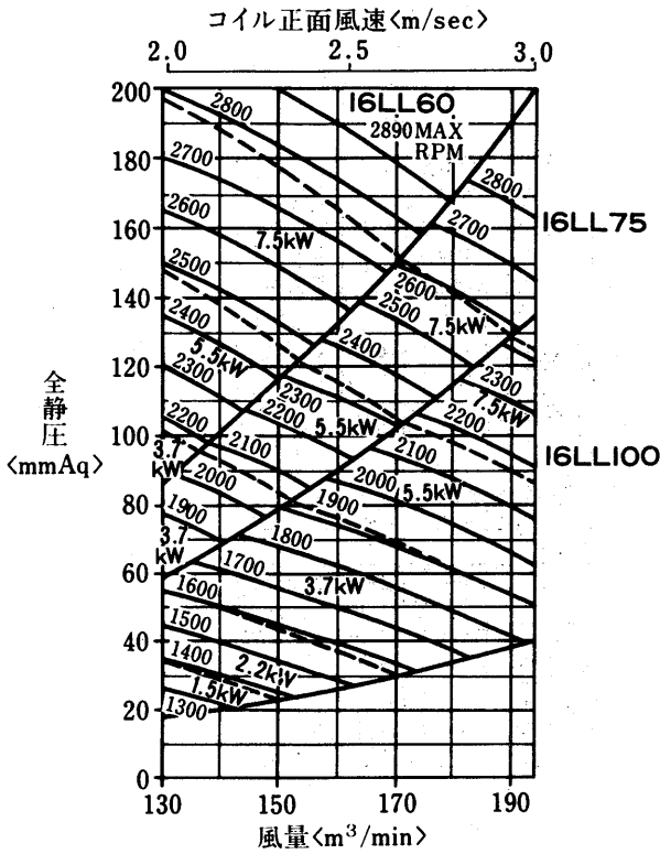
AD-180MA-V形 〈リミットロード(LL)ファン〉
