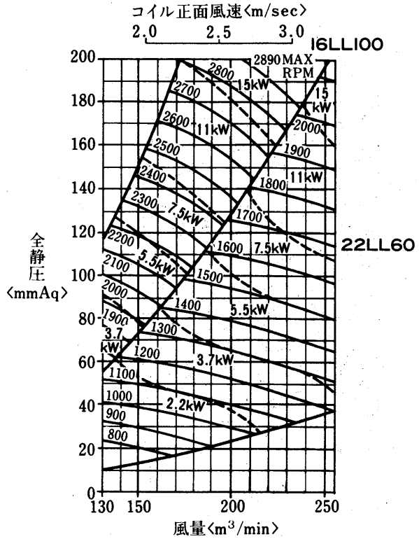
AD-200MA-V形 〈リミットロード(LL)ファン〉
