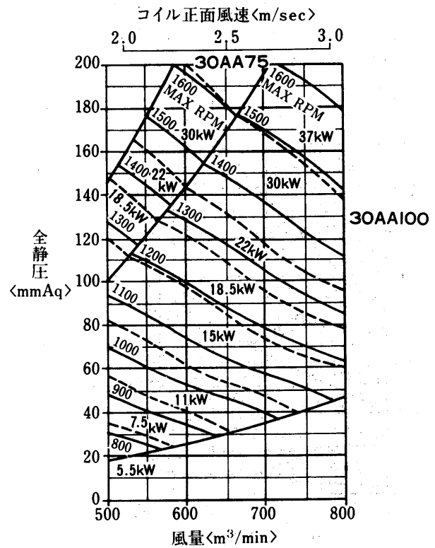
AD-700MA-H形 <エアホイル(AA)ファン>
