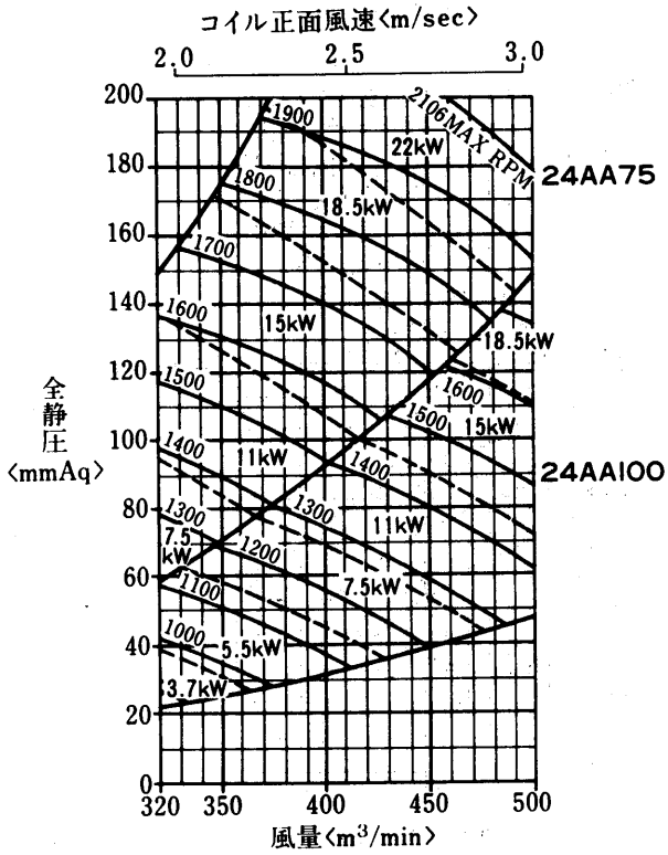
AD-450MA-H形 <エアホイル(AA)ファン>
