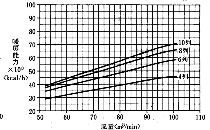
温水コイル選定図 (温水60°C)
