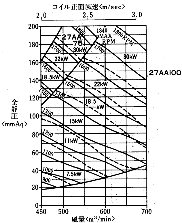
AD-600MA-H形 <エアホイル(AA)ファン>
