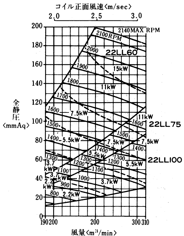
AD-270MA-V形 〈リミットロード(LL)ファン〉
