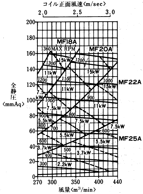
AD-380MA-V形 〈シロッコI連ファン〉
