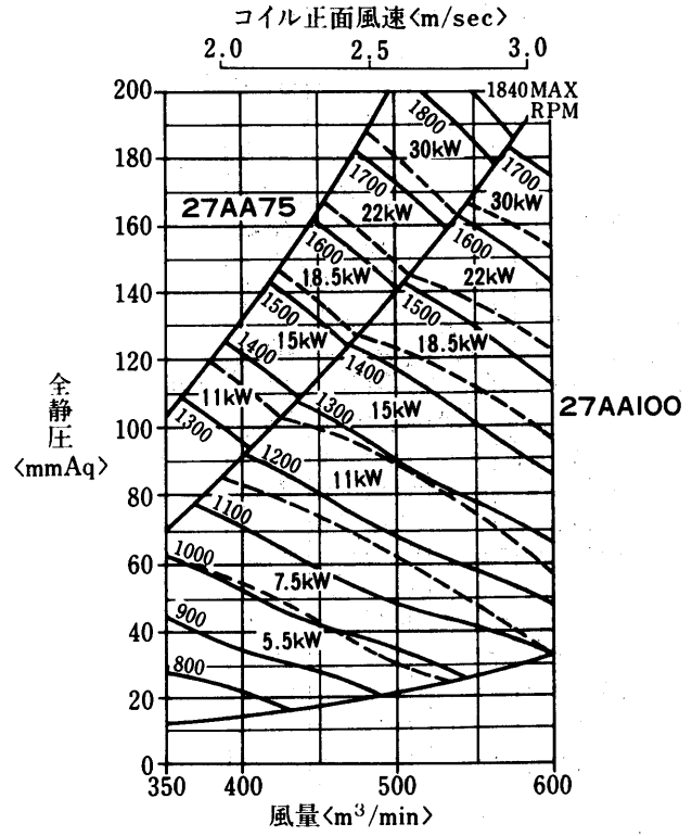
AD-530MA-H形 <エアホイル(AA)ファン>
