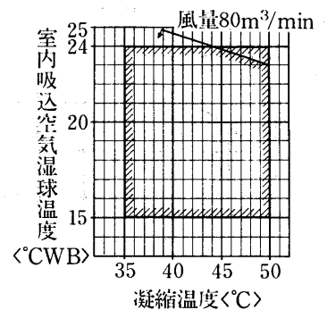
運転温度範囲
