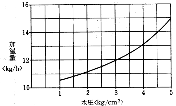
温水加湿器能力線図<別売部品>
