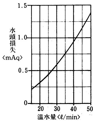
水頭損失線図
