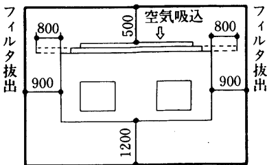
PW-40・50E形 サービススペース
