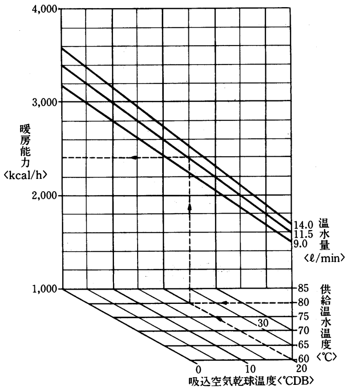
温水加熱器能力線図
