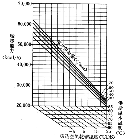
温水加熱器能力線図<2列20段><別売部品>
