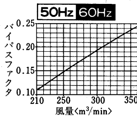
凝縮器特性線図
