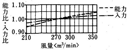
風量補正線図
