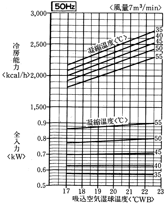
MGL-25SD-〈L〉形 冷房能力線図 MGL-25TD 1 -〈L〉形
