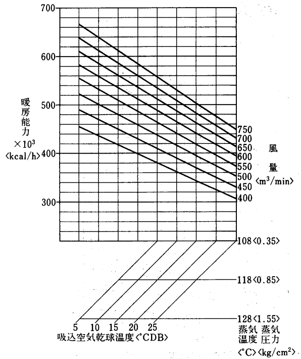
蒸気加熱器能力線図<2列><別売部品>
