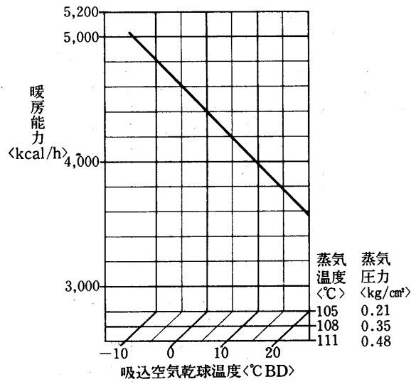
蒸気加熱器能力線図
