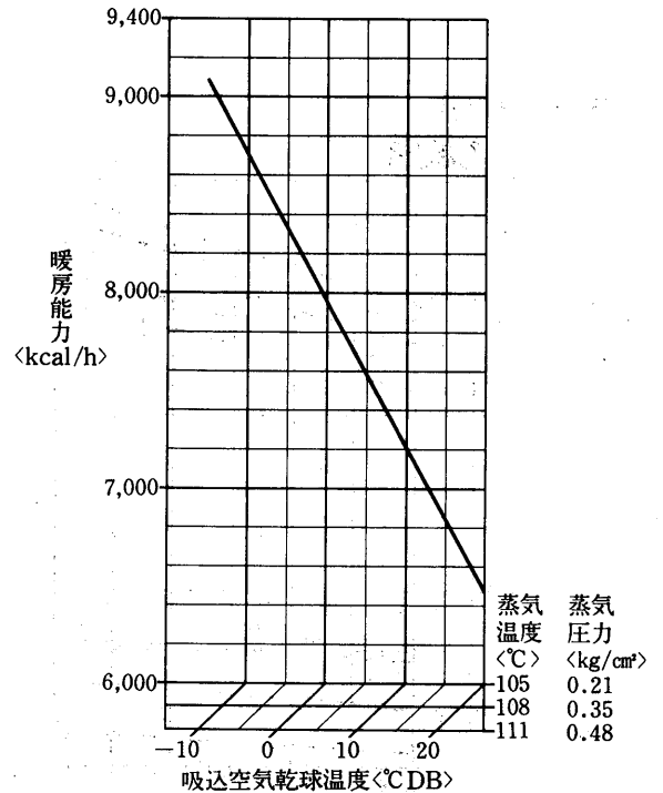
蒸気加熱器能力線図
