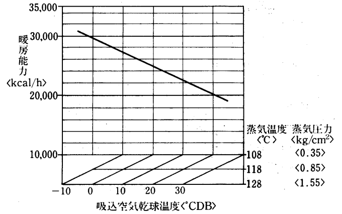
蒸気加熱器能力線図<2列×14段><別売部品>
