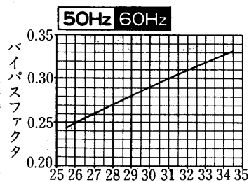
バイパスファクタ線図
