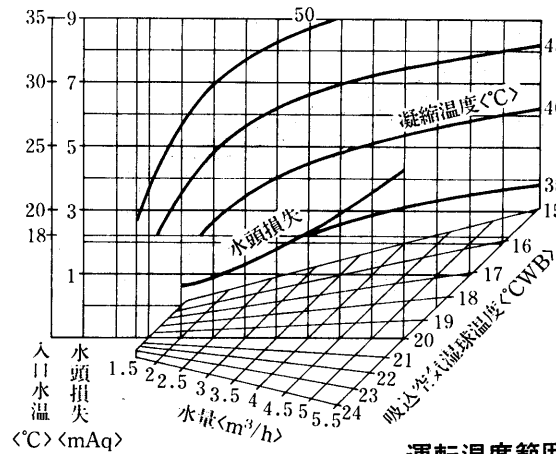
運転温度範囲
