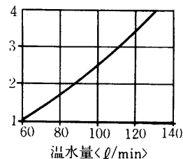
水頭損失線図
