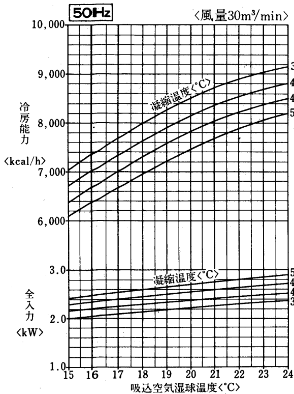
MB-90TB形 冷房能力線図
