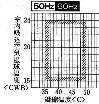
運転温度範囲
