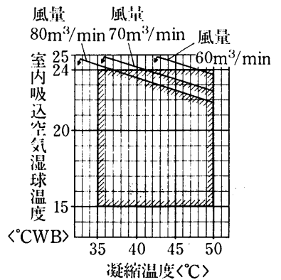
運転温度範囲
