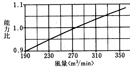
温水加湿器能力線図<別売部品>
