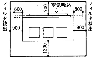
PW-60・80E形 サービススペース
