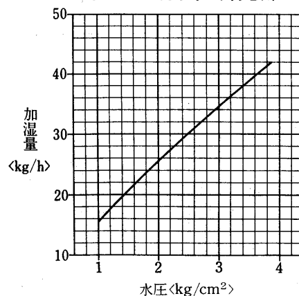
水加湿器能力線図<別売部品>
