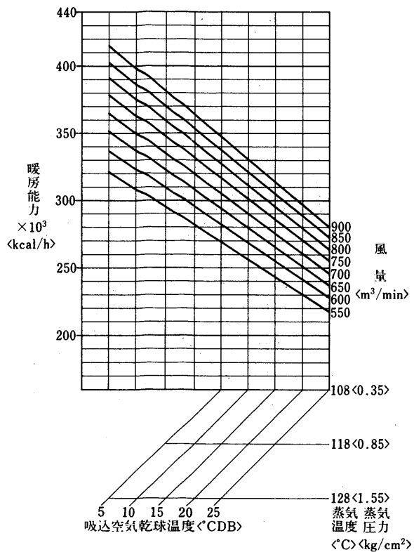
蒸気加熱器能力線図<1列><別売部品>
