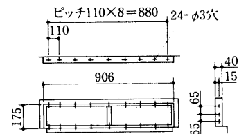
吹出ダクトフランジ <別売部品>
