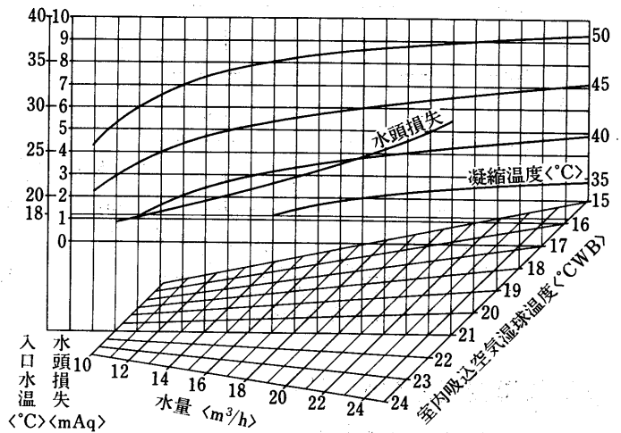
凝縮器特性線図
