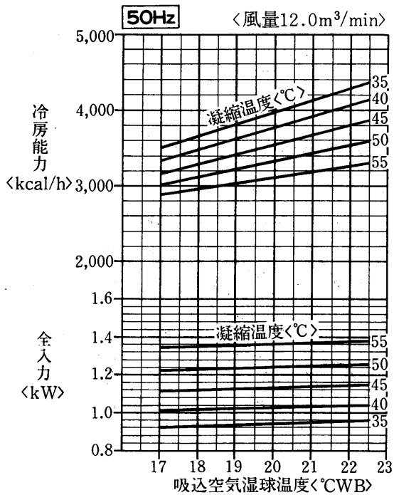
MGL-40TD 1 -<L>形冷房能力線図
