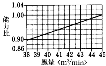
風量補正線図
