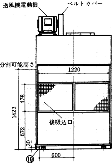
後吸込ダクトフランジ 〈別売部品〉 〈ダクト押え付〉
