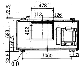
外気取入フランジ 〈別売部品〉 〈135〉
