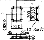
外気取入フランジ 〈別売部品〉 〈135〉
