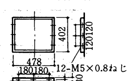
吹出ダクトフランジ 〈ダクト押え付〉
