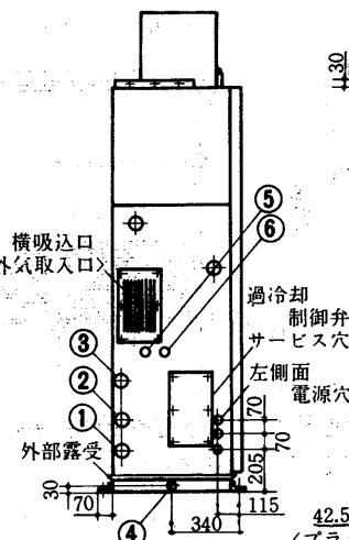
外気取入フランジ 〈別売部品〉 〈135〉
