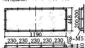
後吸込ダクトフランジ 〈別売部品〉〈ダクト押え付〉
