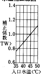
水温補正線図
