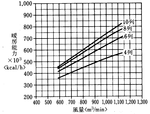
温水コイル選定図 <温水60°C>
