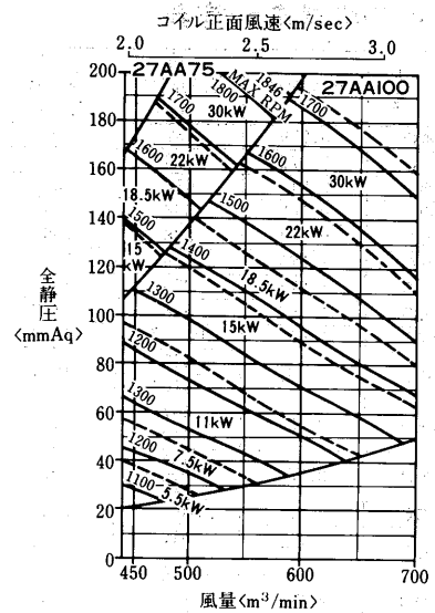
AD-600MA 2 -V形 <エアホイル(AA)ファン>
