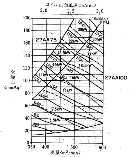
AD-800MA 2 -H形 <エアホイル(AA)ファン>
