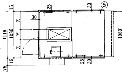
コイル配管位置寸法 <シングルフロー>
