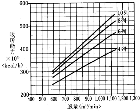
温水コイル選定図 <温水45°C>
