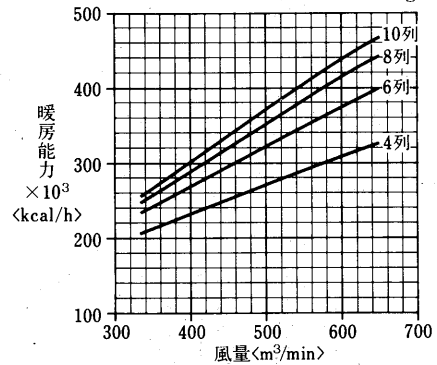
温水コイル選定図 <温水60°C>
