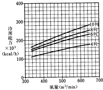
冷水コイル選定図
