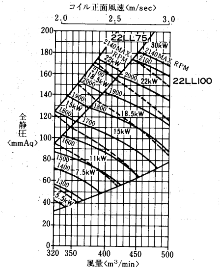
AD-450MA 2 -V形 <リミットロード(LL)ファン>
