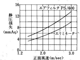
フィルタ、エリミネータの静圧損失
