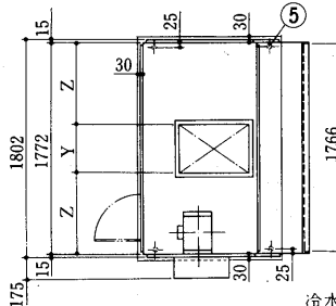
コイル配管位置寸法 (シングルフロー)
