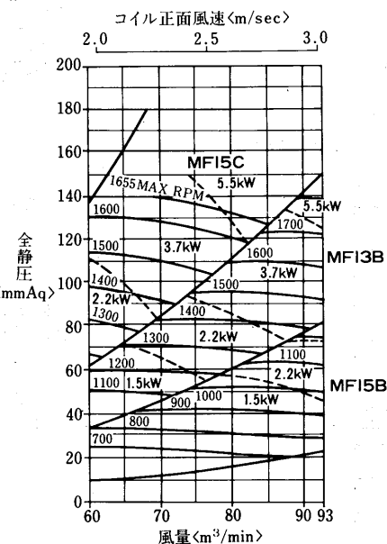
縦形シロッコファン
