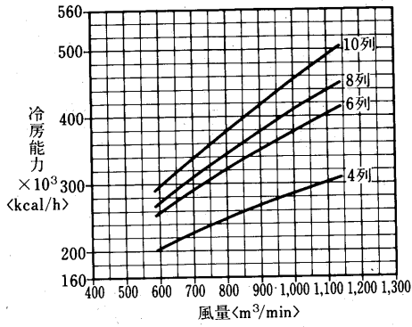
冷水コイル選定図
