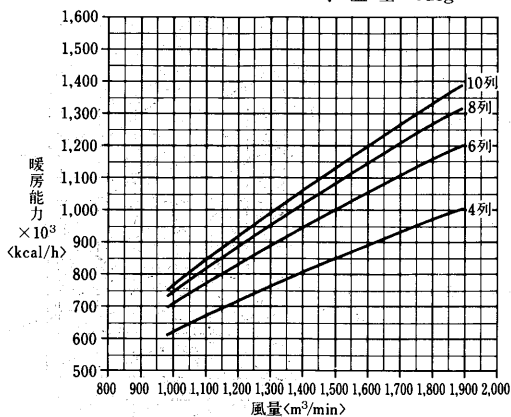
温水コイル選定図 〈温水45℃〉
