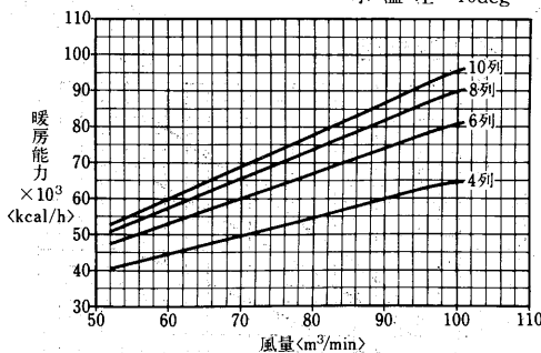
温水コイル選定図 〈温水60°C〉
