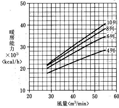
温水コイル選定図 〈温水45°C〉
