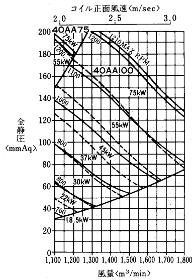
AD-180MA 2 -V形 <リミットロード(LL)ファン>
