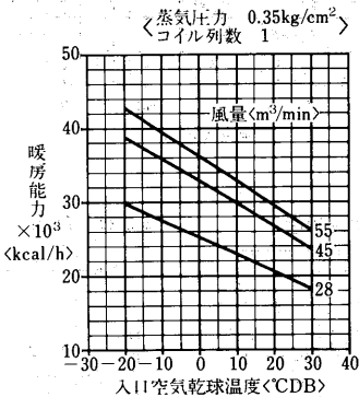
蒸気加熱コイル能力線図
