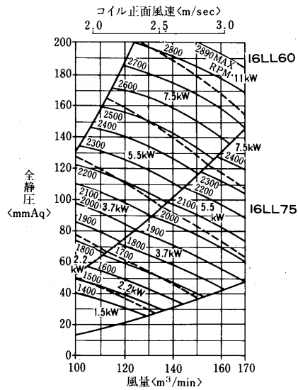
AD-240MA 2 -V形 <リミットロード(LL)ファン>
