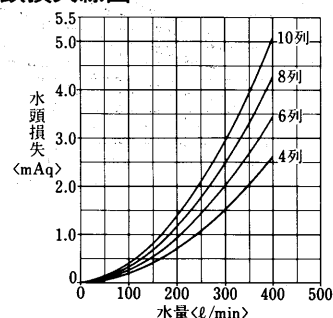
水頭損失線図
