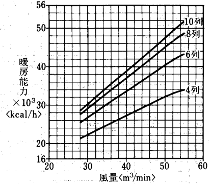
温水コイル選定図 〈温水60°C〉
