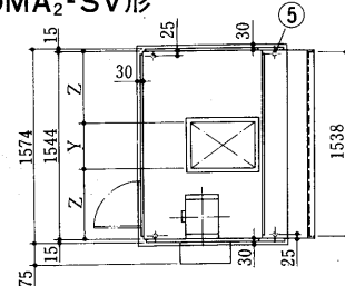
コイル配管位置寸法 (シングルフロー)
