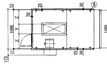
コイル配管位置寸法 <シングルフロー>
