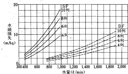
水頭損失線図
