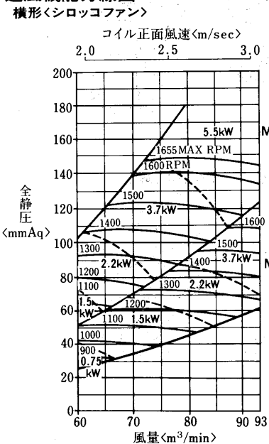
送風機能力線図
