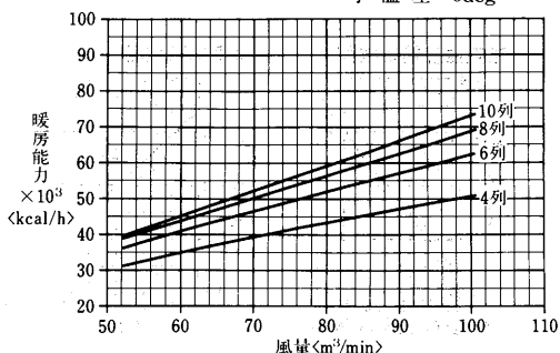
温水コイル選定図 〈温水45°C〉
