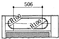
トラック状吹出ダクトフランジ<別売部品> 取付の場合
