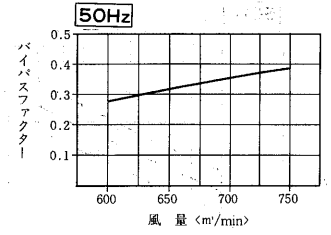
バイパスファクター線図
