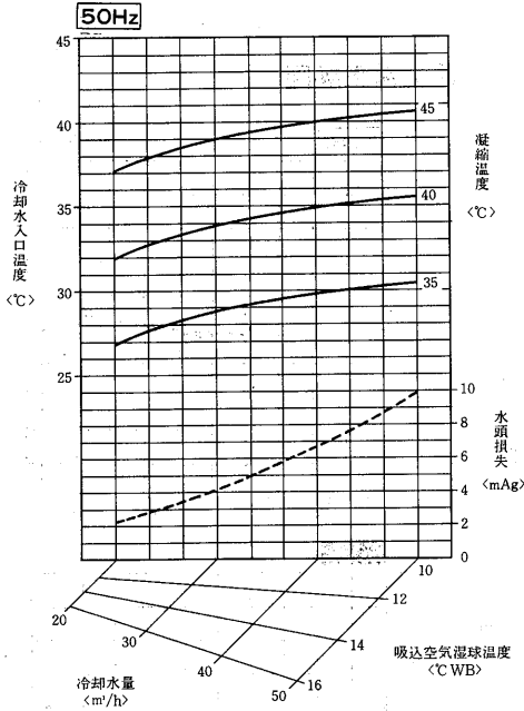
凝縮器特性線図
