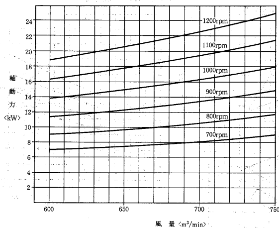
送風機性能線図
