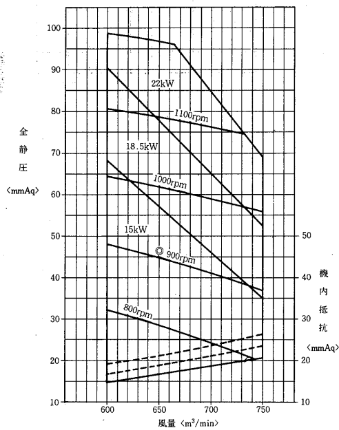
送風機軸動力線図
