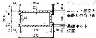
ユニット底面寸法図
