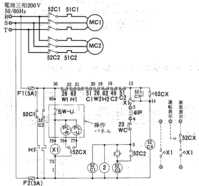
BCL-15形
