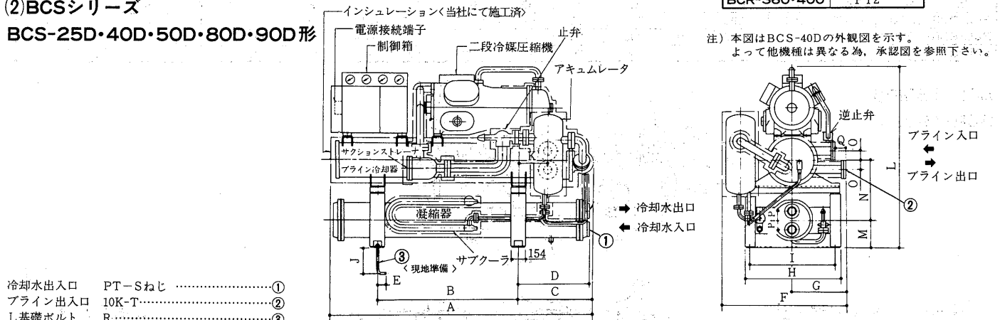
変化寸法表
