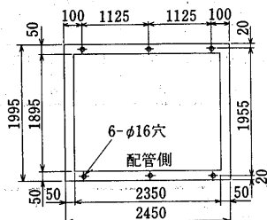
BAL-40G形
