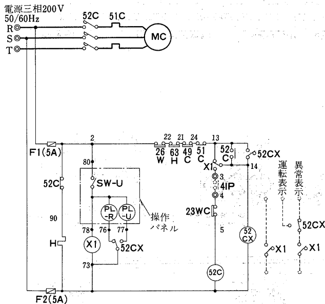
BCL-10形
