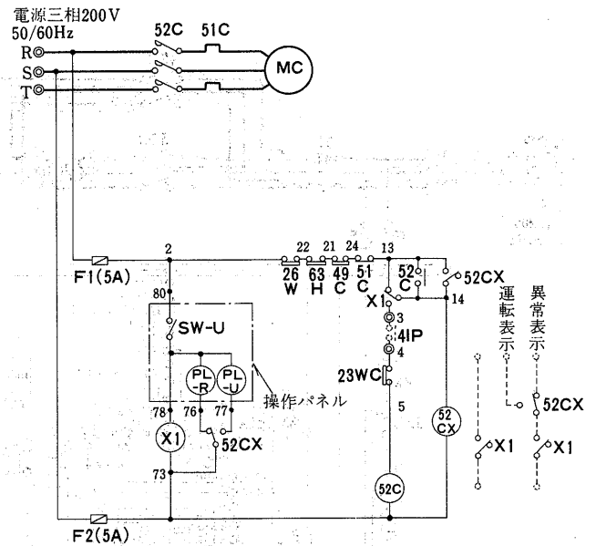
BCL-15形
