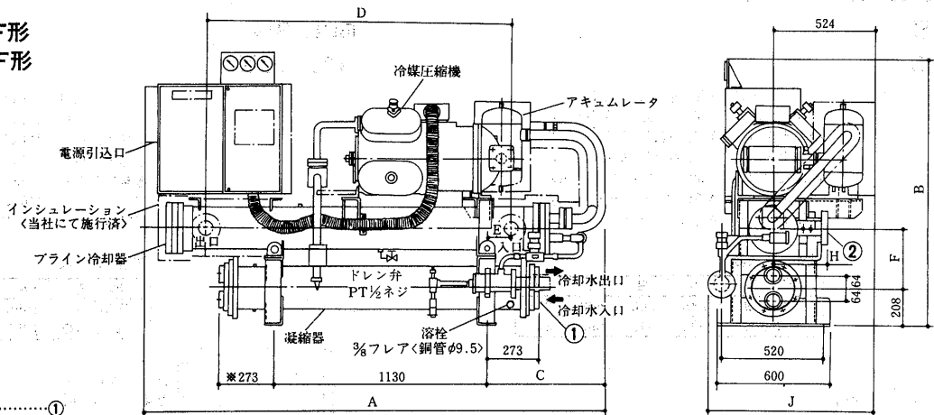
変化寸法表
