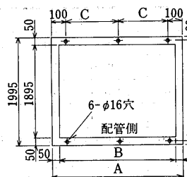
BAL-50G・60G形
