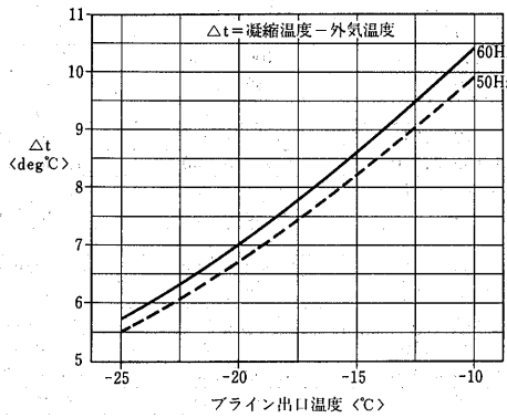
BFR形 <第2図>
