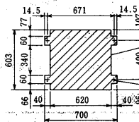
ユニット底面寸法図
