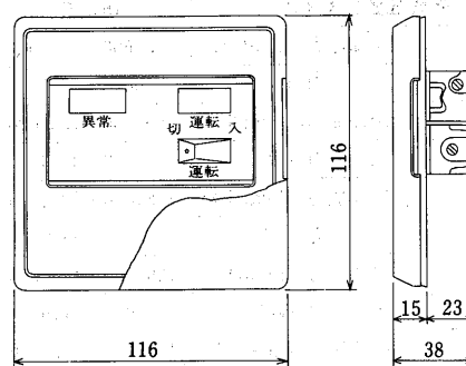
リモコンパネル寸法
