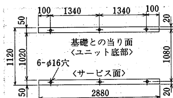
BAL-40G形
