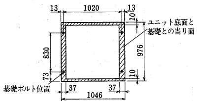
ユニット底面寸法図
