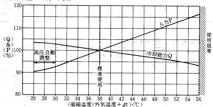
BFS形 <第5図>
