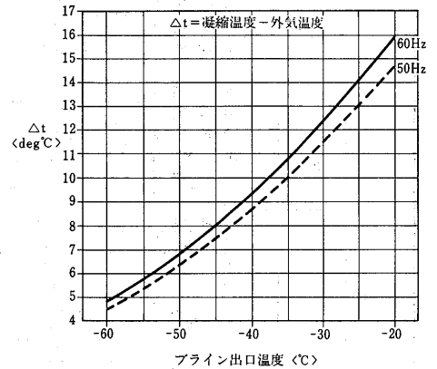
BFS形 <第3図>
