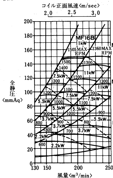
送風機能力線図 横形<シロココファン>
