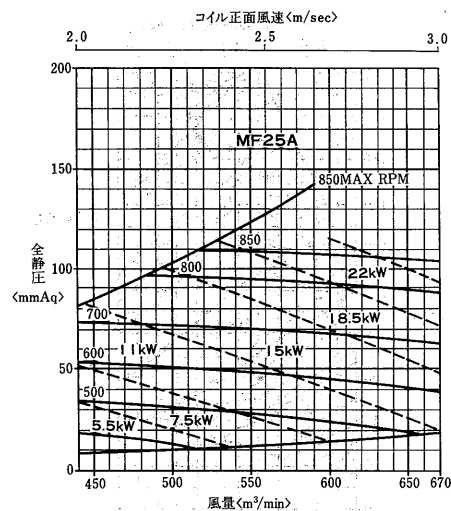
AD-60OMA 2 -H形 <シロッコ(MF)ファン>
