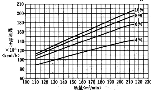
温水コイル選定図 〈温水60°C〉
