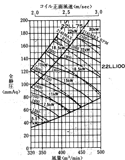
AD-45OMA 2 -H形 <リミットロード(LL)ファン>
