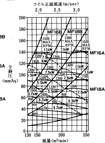
縦形<シロココファン>
