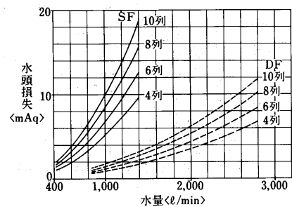
水頭損失線図
