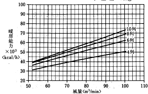
温水コイル選定図 〈温水45°C〉
