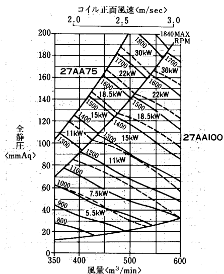
AD-53OMA 2 -H形 <エアホイル(AA)ファン>
