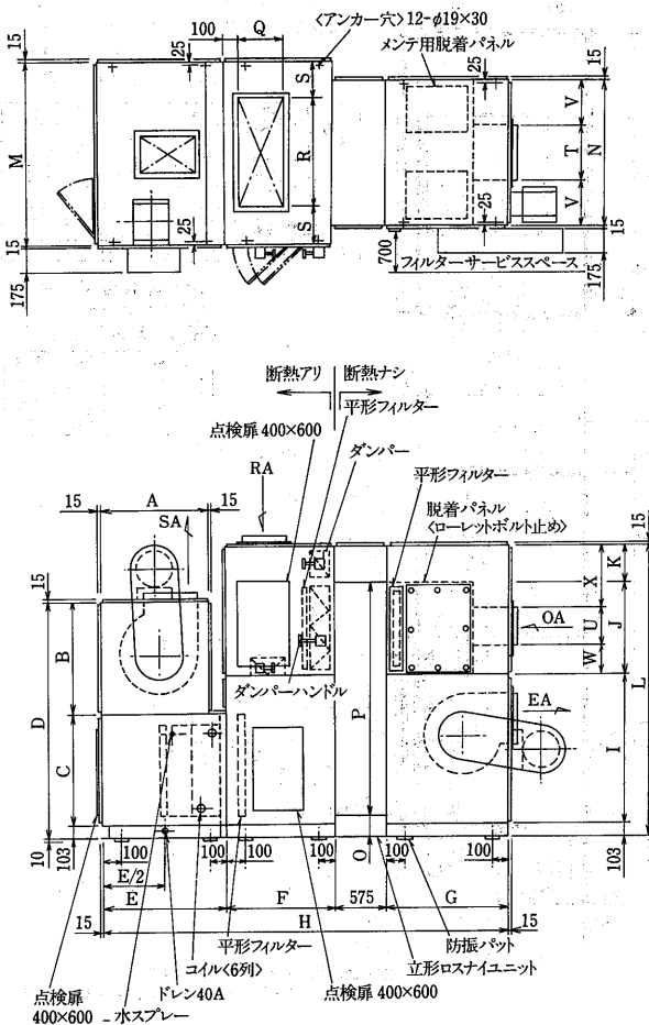
変化寸法表
