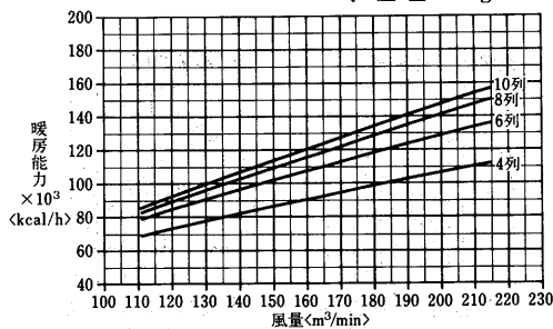
温水コイル選定図 〈温水45°C〉
