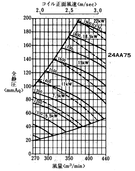
AD-530MA 2 -V形 <エアホイル(AA)ファン>
