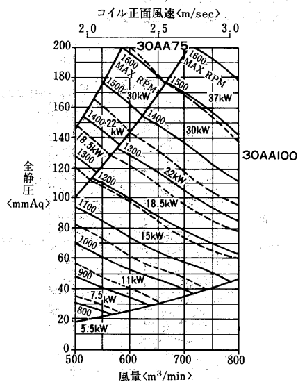
AD-70OMA 2 -H形 <エアホイル(AA)ファン>
