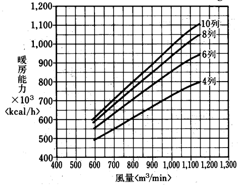
温水コイル選定図 〈温水60°C〉
