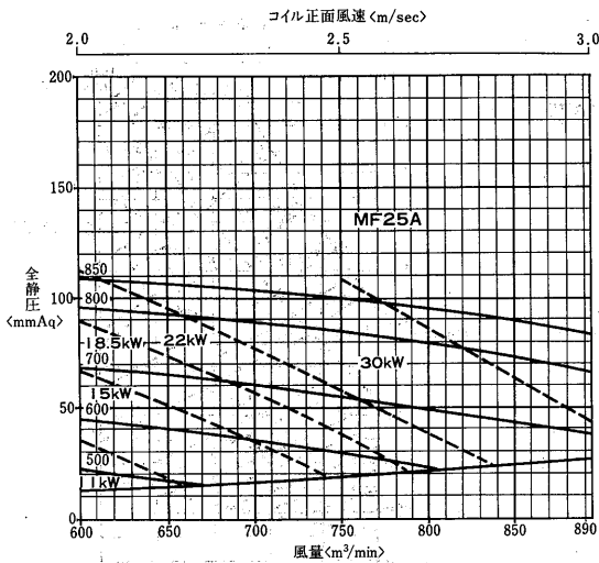
AD-800MA 2 -V形 <シロッコ(MF)ファン>
