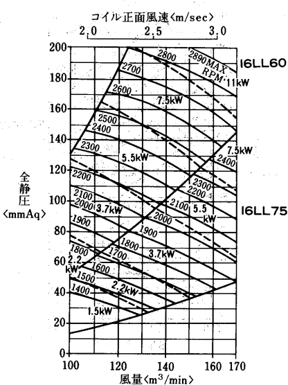
AD-150MA 2 -V形 〈リミットロード(LL)ファン〉
