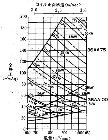
AD-1400MA 2 -H形 〈エアホイール(AA)ファン〉
