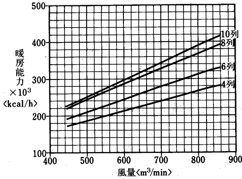
温水コイル選定図 <温水45°C>
