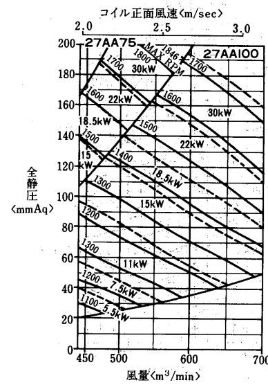
AD-700MA 2 -V形 <シロッコ(MF)ファン>
