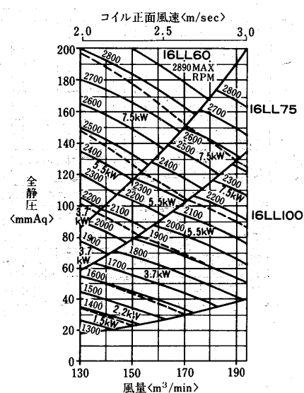
AD-180MA 2 -V形 〈リミットロード(LL)ファン〉
