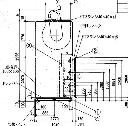
コイル配管位置寸法<シングルフロー>
