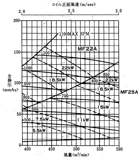
AD-530MA 2 -V形 <シロッコ(MF)ファン>
