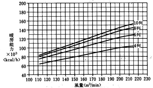
温水コイル選定図 <温水60°C>
