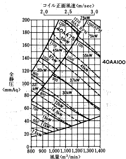
AD-1200MA 2 -H形 〈エアホイール(AA)ファン〉
