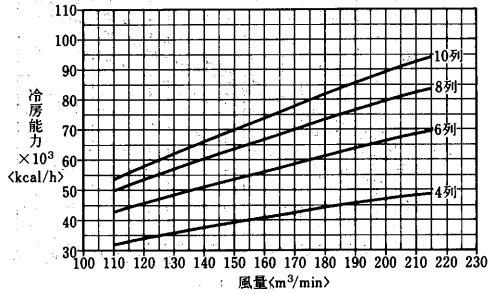
冷水コイル選定図
