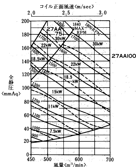
AD-70OMA 2 -H形 <エアホイル(AA)ファン>
