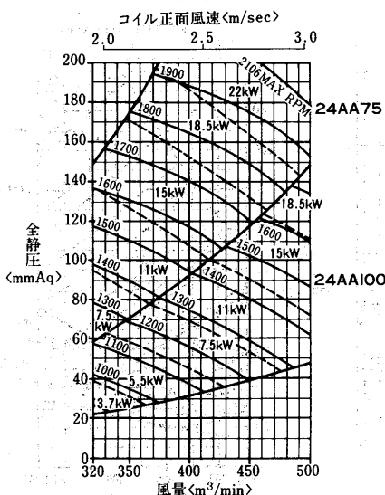
AD-45OMA 2 -H形 <エアホイル(AA)ファン>
