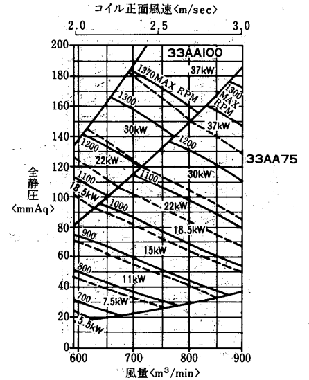
AD-800MA 2 -V形 <エアホイール(AA)ファン>
