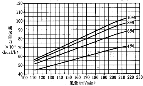
温水コイル選定図 <温水45°C>
