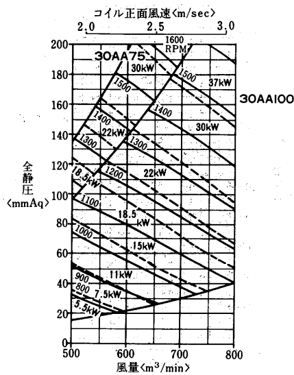
AD-800MA 2 -V形 <シロッコ(MF)ファン>
