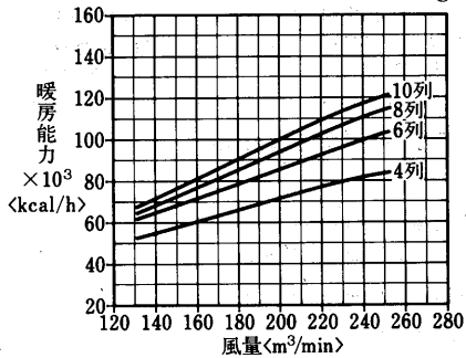
温水コイル選定図 <温水45°C>
