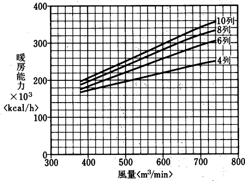
温水コイル選定図 <温水45°C>
