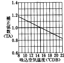
空気温度補正線図
