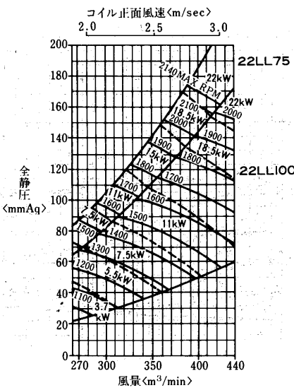
AD-450MA 2 -V形 <エアホイル(AA)ファン>
