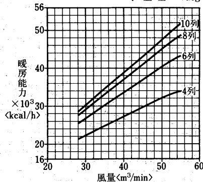
温水コイル選定図 〈温水60℃〉
