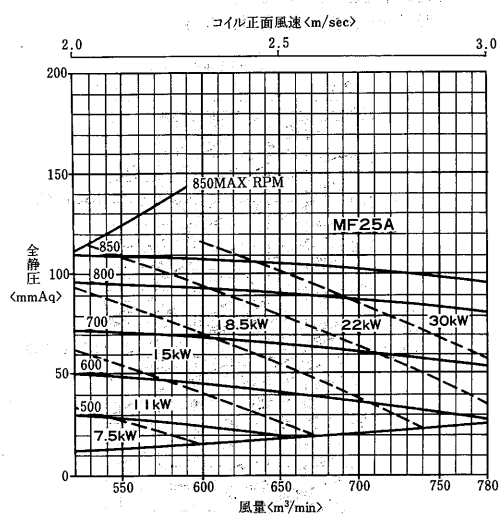
AD-70OMA 2 -H形 <シロッコ(MF)ファン>
