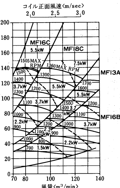
縦形<シロッコファン>
