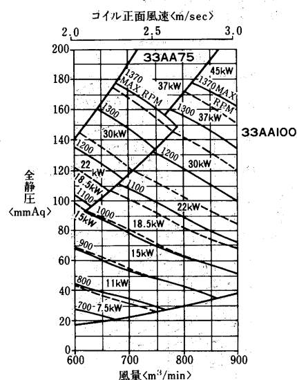
AD-80OMA 2 -H形 <エアホイル(AA)ファン>
