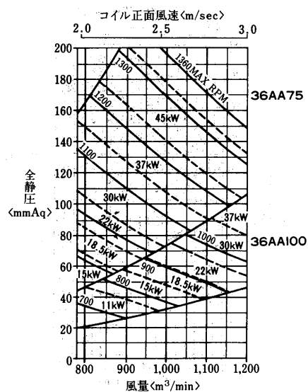
AD-1500MA 2 -H形 〈エアホイール(AA)ファン〉
