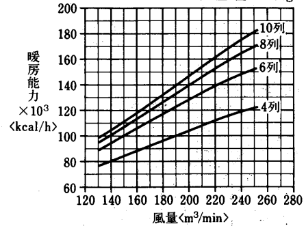
温水コイル選定図 <温水60°C>
