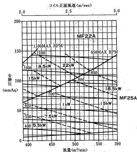
AD-53OMA 2 -H形 <シロッコ(MF)ファン>
