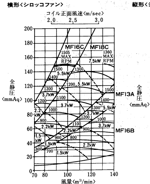
送風機能力線図
