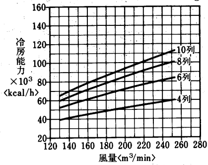
冷水コイル選定図
