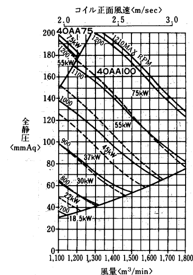
AD-1500MA 2 -H形 〈エアホイール(AA)ファン〉
