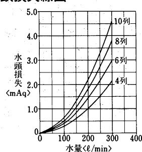
水頭損失線図
