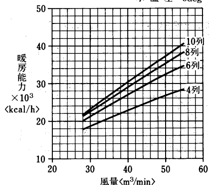
温水コイル選定図 〈温水45℃〉
