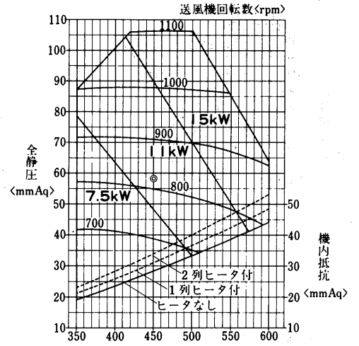
送風機性能線図
