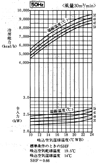
冷房能力線図
