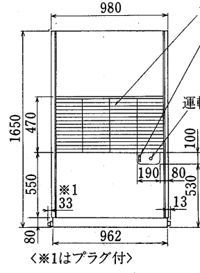
分ダクト穴詳細図
