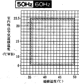
運転温度範囲
