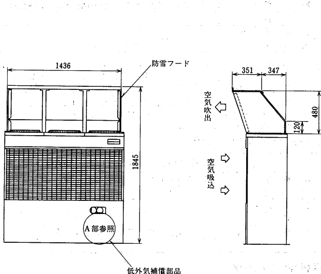
A部詳細図<PUTF(S)-8・10A>
