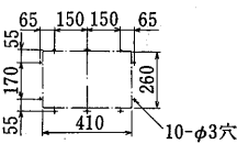
分ダクト穴詳細図
