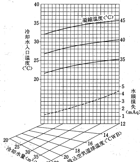
凝縮器特性線図
