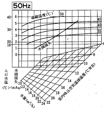
運転温度範囲
