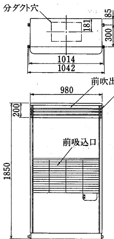
分ダクト穴詳細図
