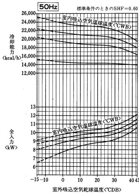
PCTS-10PLA形 冷却能力線図
