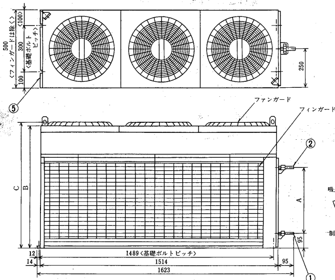
変化寸法表
