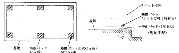
基礎図<参考>
