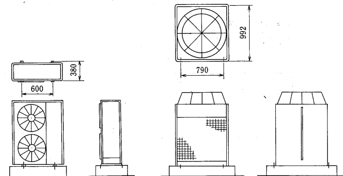
基礎図<参考>
