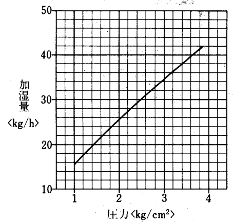
蒸気加湿器能力線図
