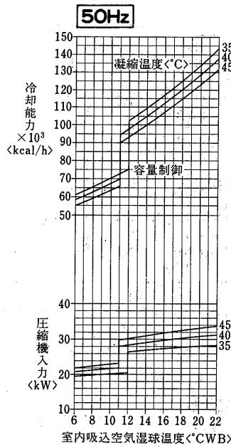
PWT-50G形 冷房能力線図
