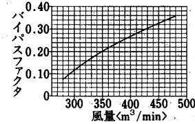
バイパスファクタ線図 60Hz
