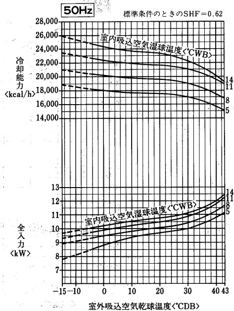
PCTF-10PLA形 冷却能力線図
