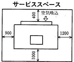
変化寸法表
