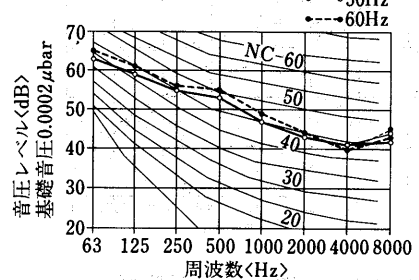
(b) 室外ユニット PUTF-5A形 PUTS-5A形
