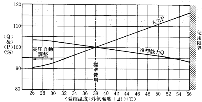
BFS形 <第5図>
