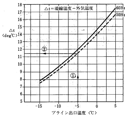
BFL形 <第1図>
