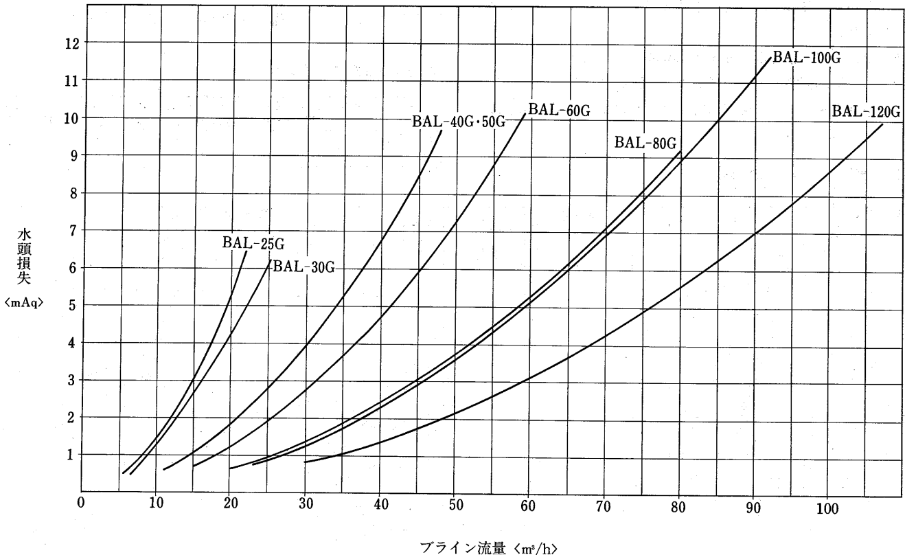
BAL-G形水頭損失曲線
