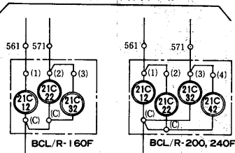
No.2 容量制御回路
