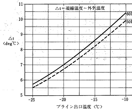
BFR形 <第2図>
