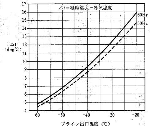
BFS形 <第3図>
