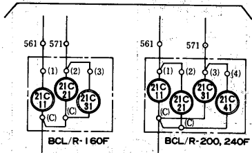
No.1 容量制御回路
