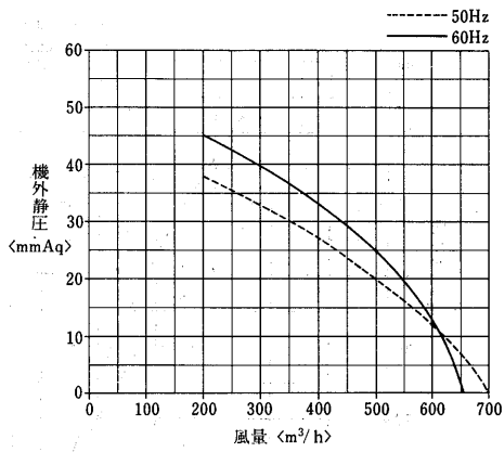
GU-500HR形
