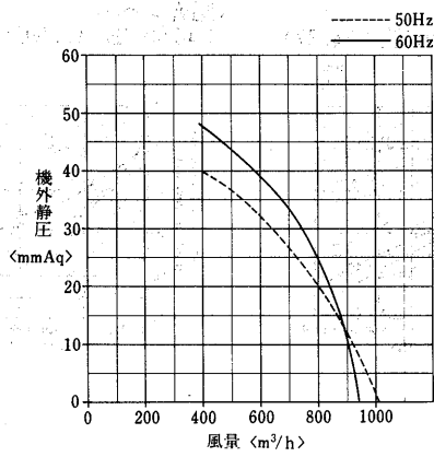
GU-800HR形
