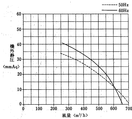
GU-500HS形
