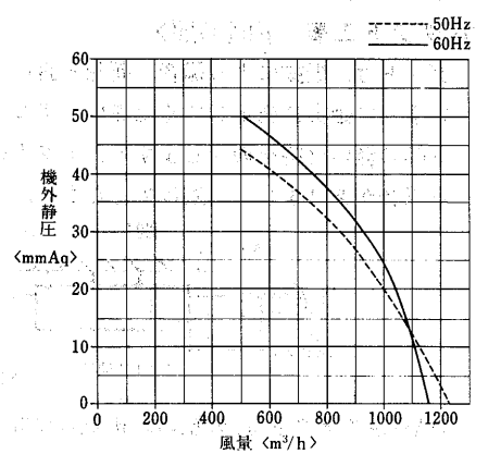
GU-1000HR形
