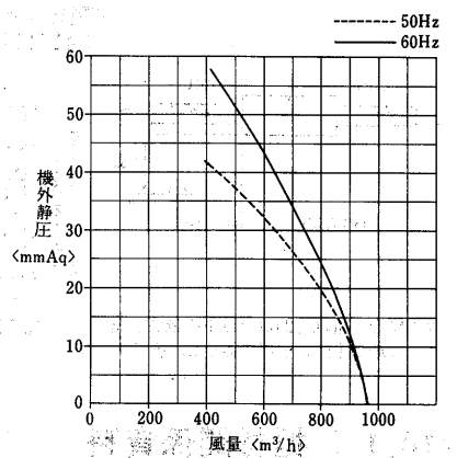
GU-800HS形
