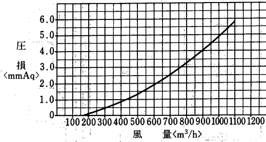
GZ-25-20D形圧力損失特性 <GU-800HR<HS>用 ダクト変換アタッチメント>
