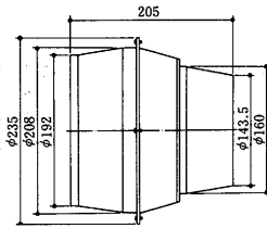
ダクト変換アタッチメント PZ-20A 2 形
