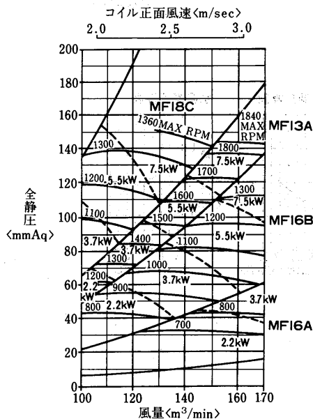
送風機能力線図
