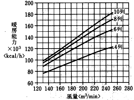
温水コイル選定図 <温水60°C>
