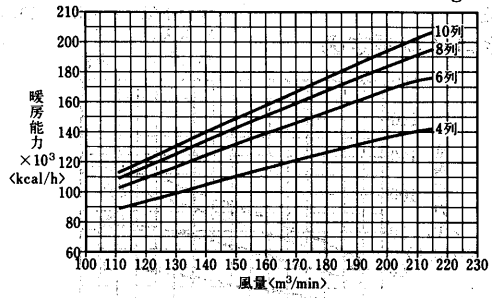
温水コイル選定図 〈温水60℃〉
