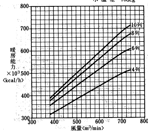
温水コイル選定図 〈温水60℃〉
