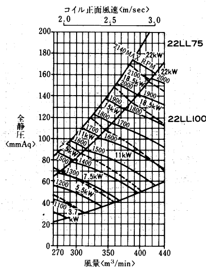
AD-380MA 2 -V形 <リミットロード(LL)ファン>
