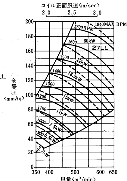
縦形<リミットロード(LL)ファン>
