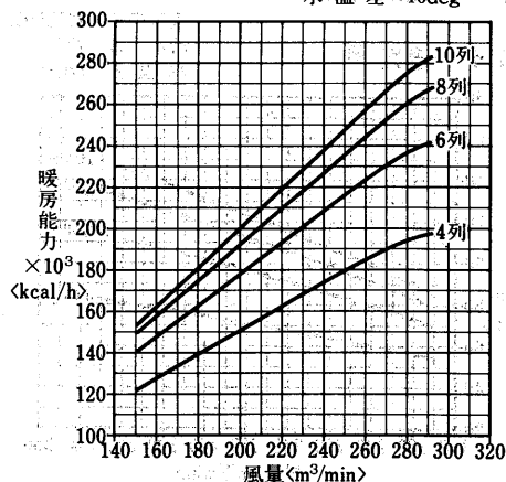
温水コイル選定図 〈温水60℃〉
