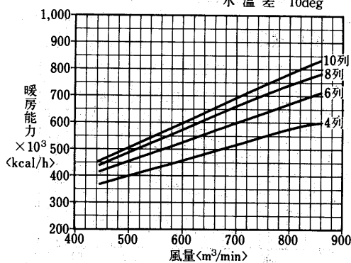
温水コイル選定図 〈温水60℃〉
