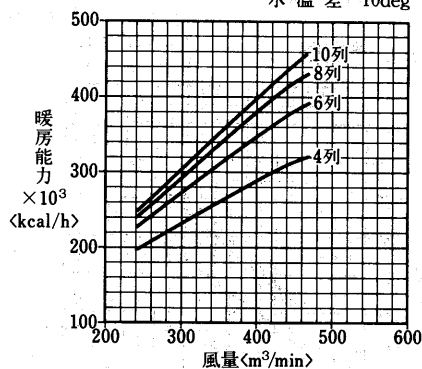
温水コイル選定図 〈温水60℃〉
