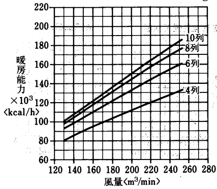
温水コイル選定図 〈温水45°C〉
