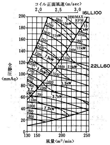
AD-300MA 2 -V形 <リミットロード(LL)ファン>
