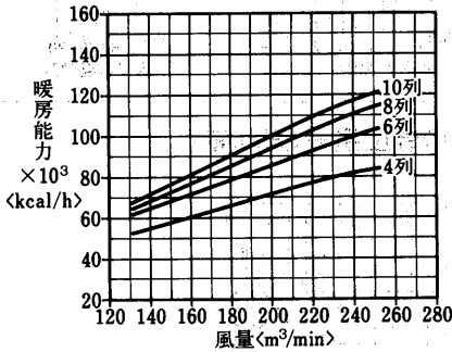
温水コイル選定図 <温水45°C>
