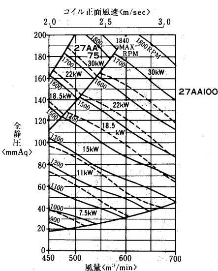
AD-600MA 2 -H形 <エアホイル(AA)ファン>
