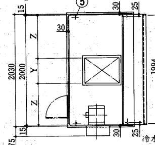
コイル配管位置寸法 (シングルフロー)
