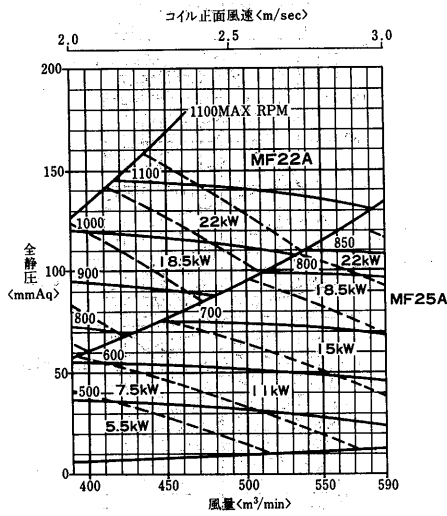
AD-530MA 2 -V形 <シロッコ(MF)ファン>
