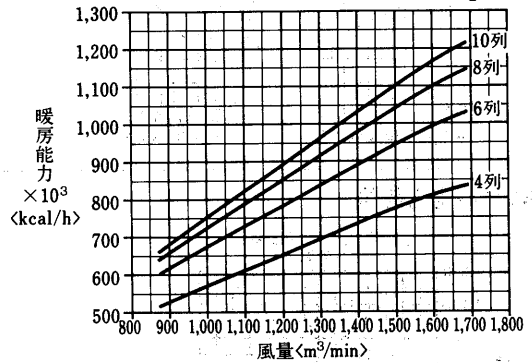
温水コイル選定図 <温水60°C>
