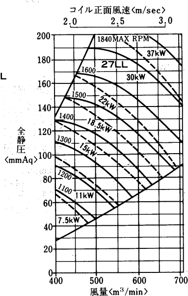
縦形クリットロード(LL)ファン
