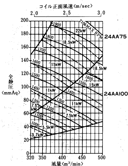
AD-450MA 2 -H形 <エアホイル(AA)ファン>
