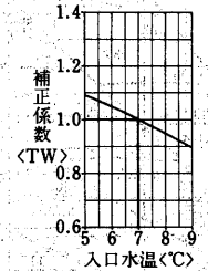
水温補正線図
