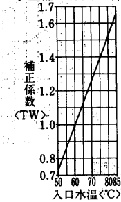
水温補正線図
