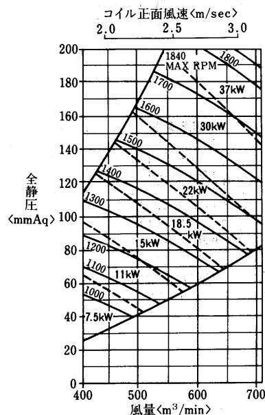
横形クリットロード(LL)ファン
