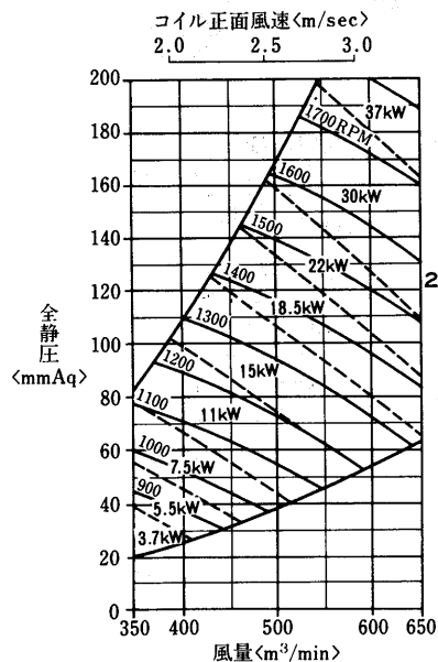
横形<リミットロード(LL)ファン>
