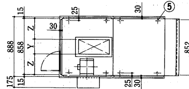
コイル配管位置寸法 <シングルフロー>
