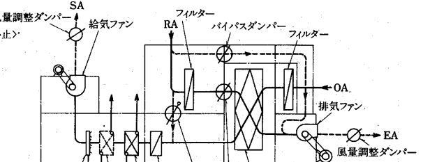
●エアフロー
