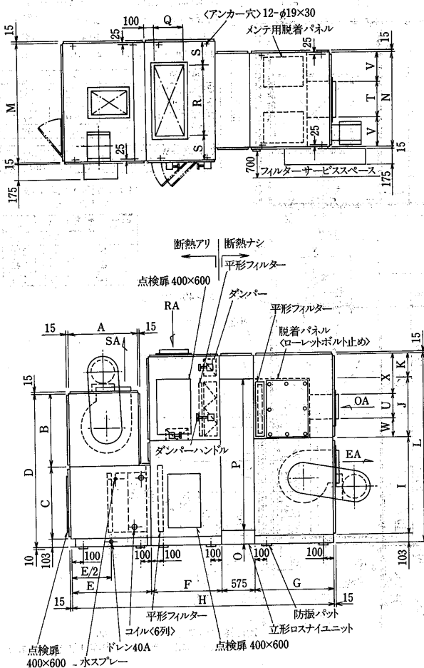
変化寸法表
