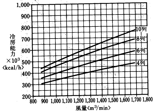
冷水コイル選定図
