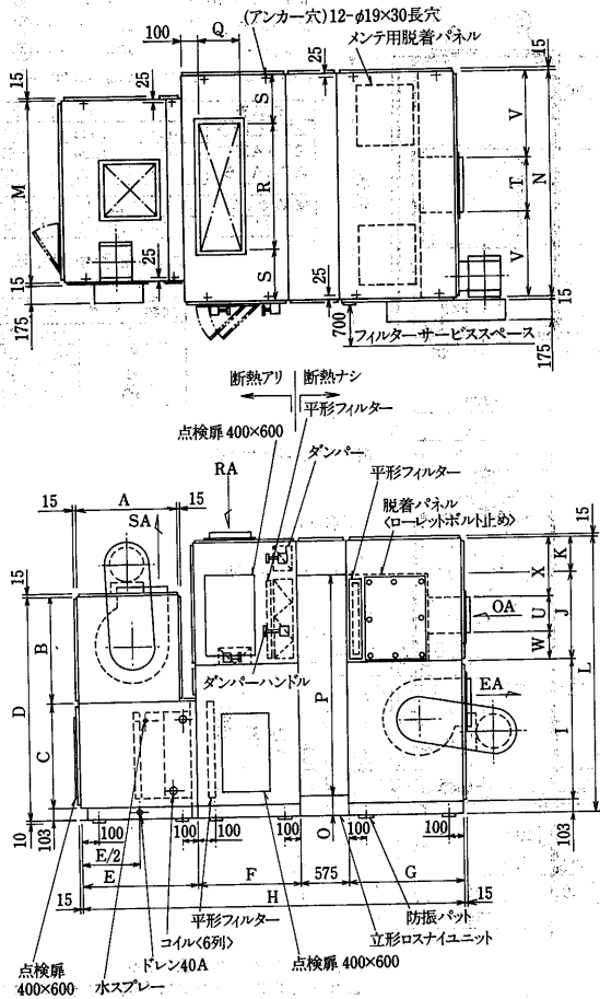
変化寸法表
