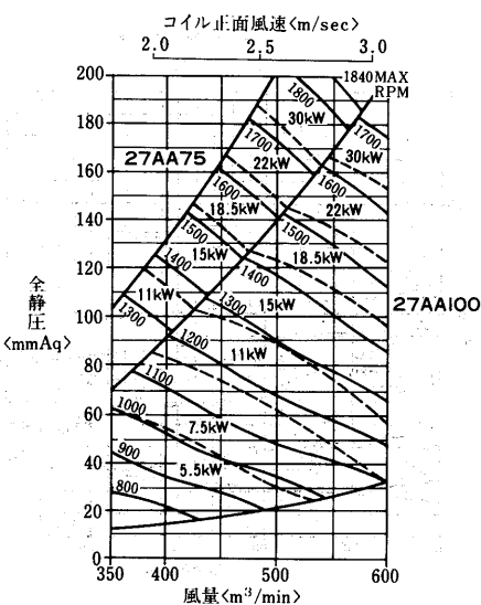
AD-530MA 2 -H形 <エアホイル(AA)ファン>
