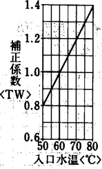
水温補正線図
