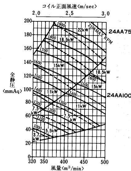
AD-450MA 2 -V形 <エアホイル(AA)ファン>
