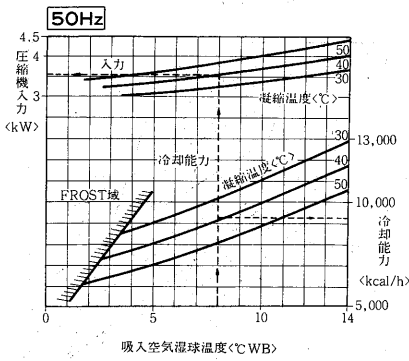
GT-50G 2 L形冷却能力線図〈風量80m 3 /min 送風機電動機1.5kW内蔵〉
