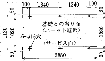
BAL-40G形
