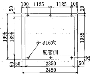
BAL-40G形
