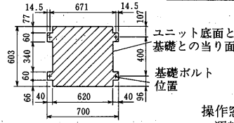
ユニット底面寸法図
