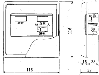
リモコンパネル寸法
