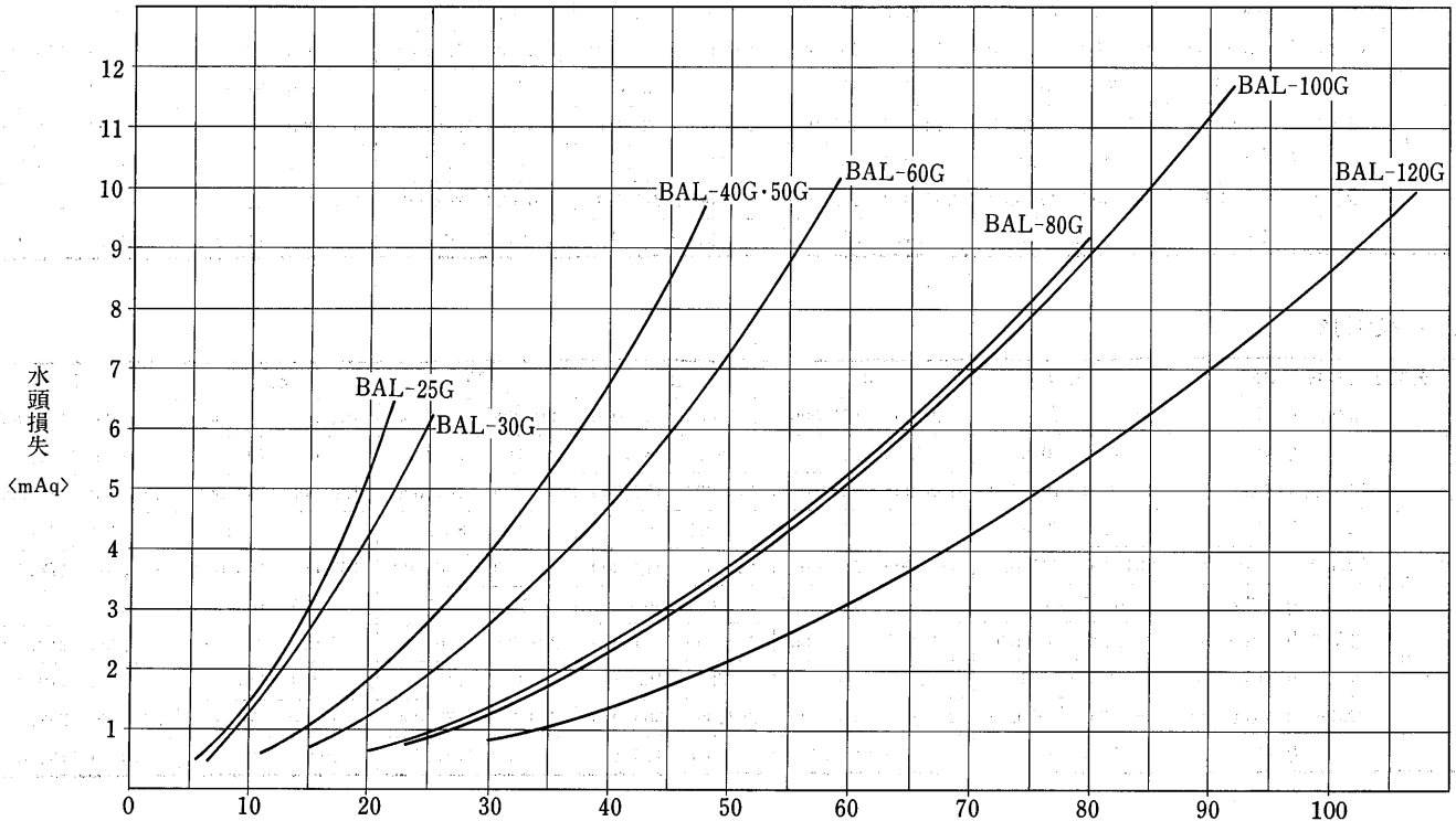
BAL-G形水頭損失曲線
