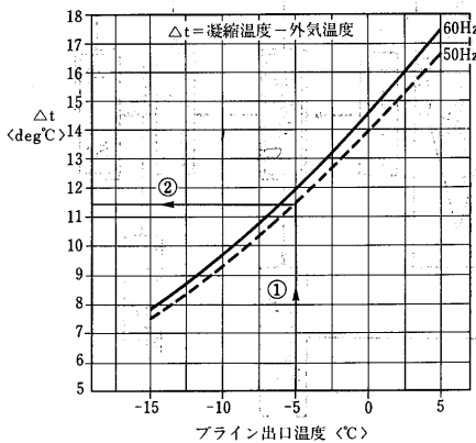
BFL形 <第1図>
