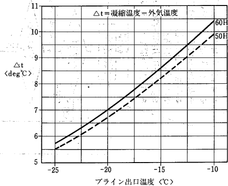
BFR形 <第2図>
