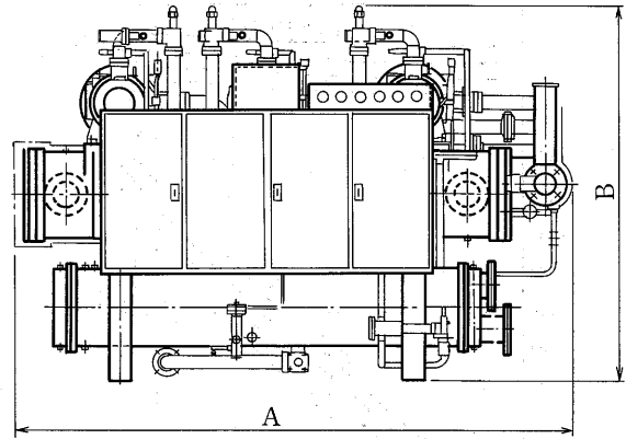
変化寸法表
