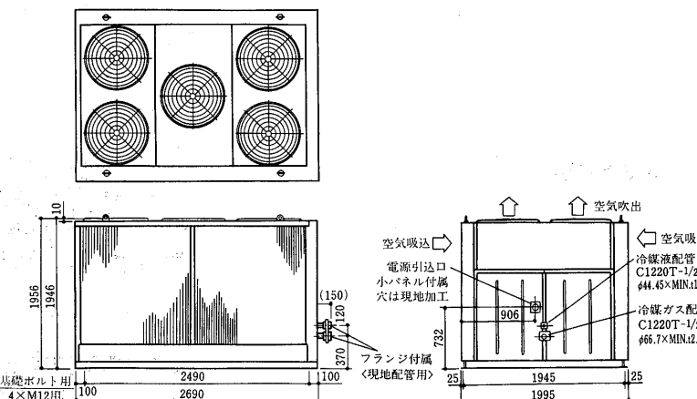
RMA-60D形
