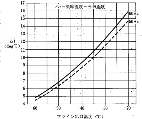
BFS形 <第3図>
