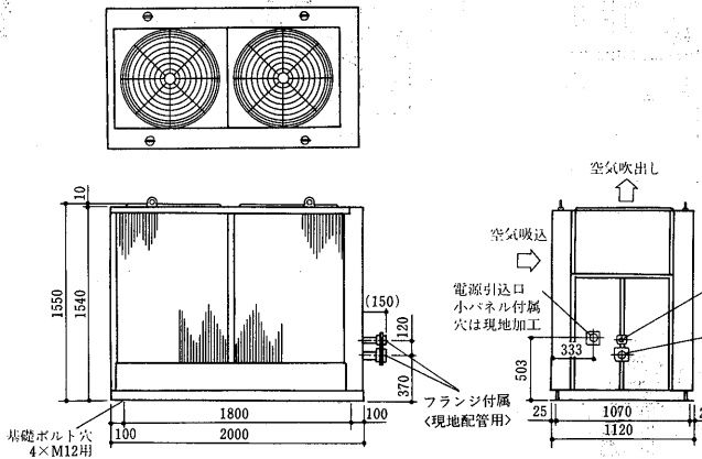
RMA-40D形
