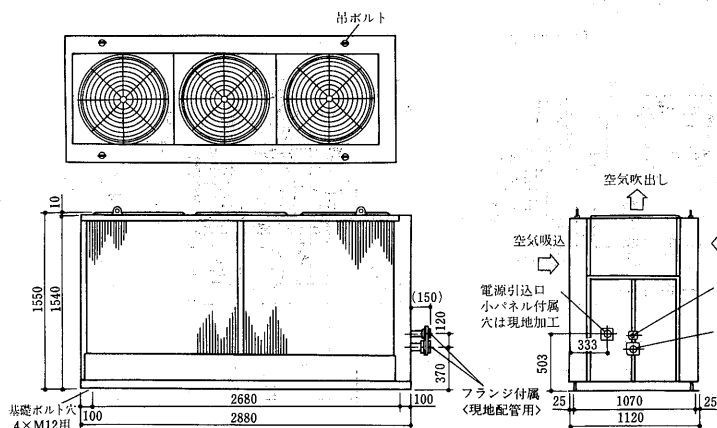
RMA-40D形
