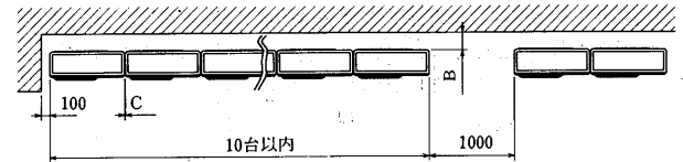
室外吹出ガイド使用時
