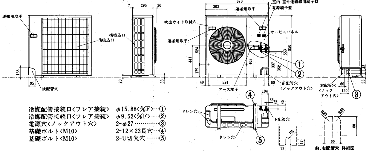
前.右配管穴 詳細図
