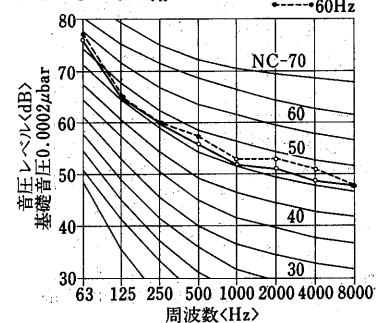
PUTS-10B形
