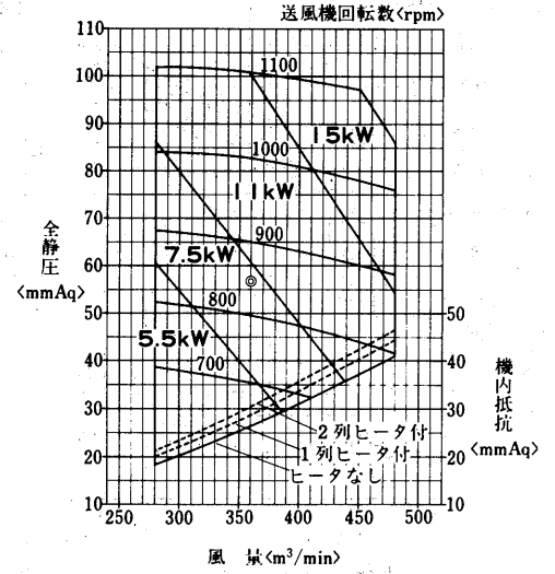
送風機軸動力線図
