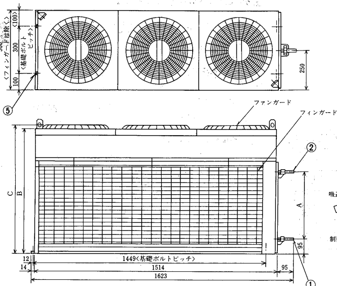
変化寸法表
