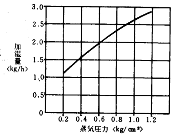
蒸気加湿器能力線図<別売部品>
