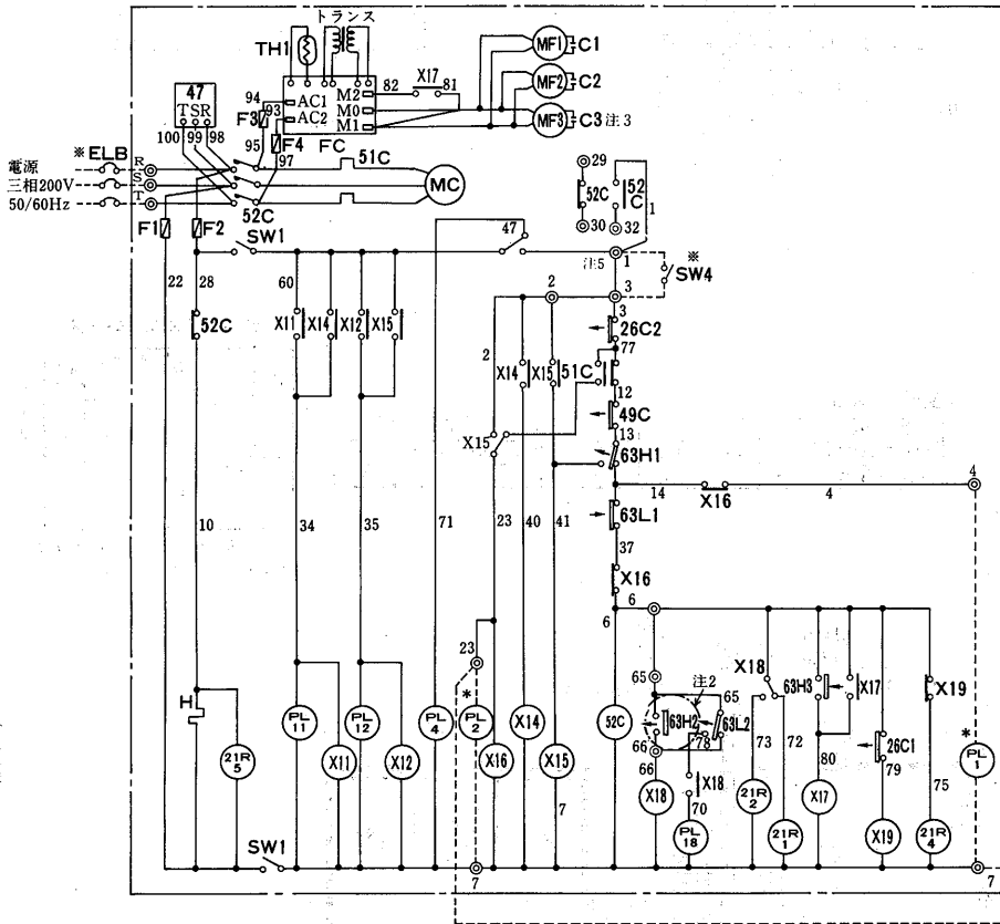
室外ユニット<PUTF-5B・8B・10B>
