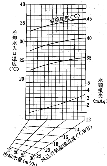
凝縮器特性線図
