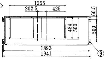
室内ユニットサービススペース
