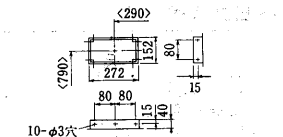
外気取入フランジ<別売部品>
