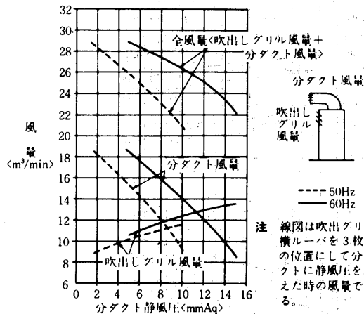
分ダクト静風圧—風量線図<Δ結線>
