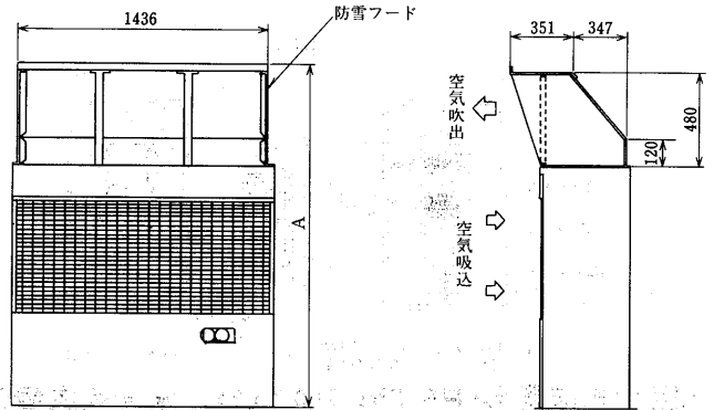
PUTF-20A形防雪フード<F-150C形> 低外気補償部品取付図
