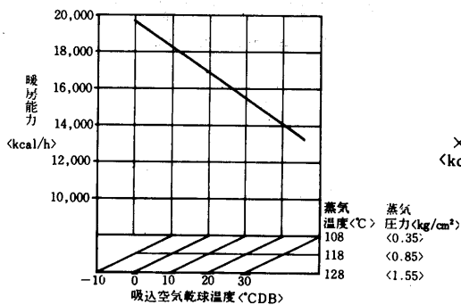
蒸気加熱器能力線図<2列×14段><別売部品>
