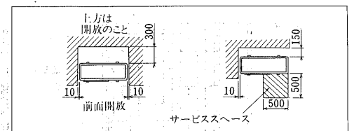
室外ユニットサービススペース
