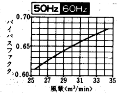
バイパスファクタ線図
