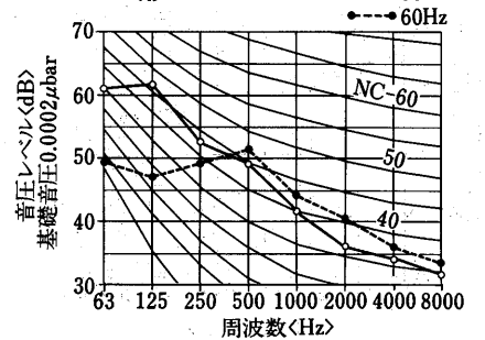
PUTS-10B形
