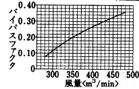
バイパスファクタ線図
