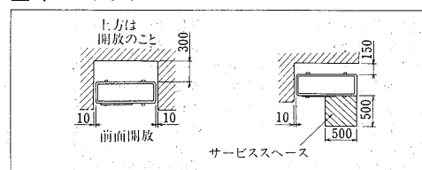
室外ユニットサービススペース
