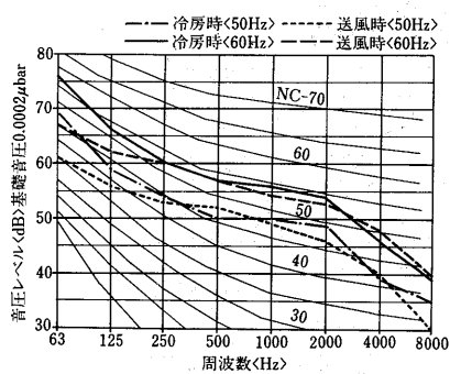
PAT-25E形 50Hz
