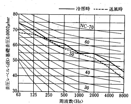
PAT-30E形 50Hz
