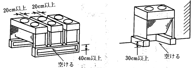
PVT-40J形
