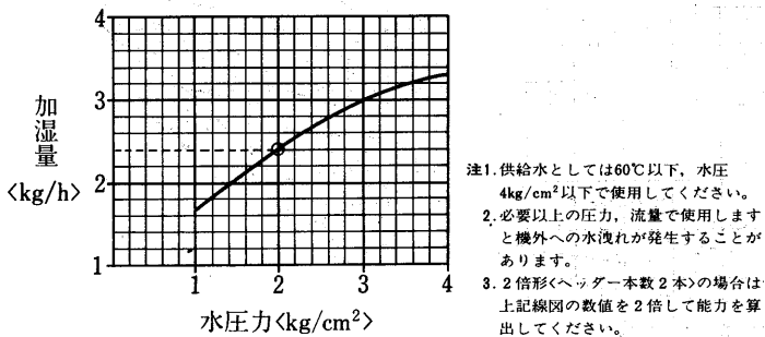
温水加湿器能力線図<別売部品>
