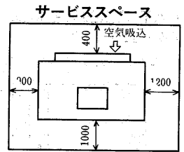
変化寸法表
