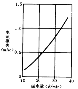
水頭損失線図
