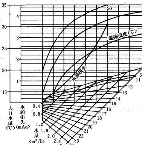
凝縮器特性線図
