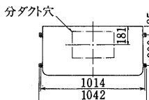
分ダクト穴詳細図
