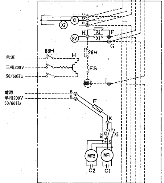
室内ユニット<PCT-2PA・3PA・4PA>
