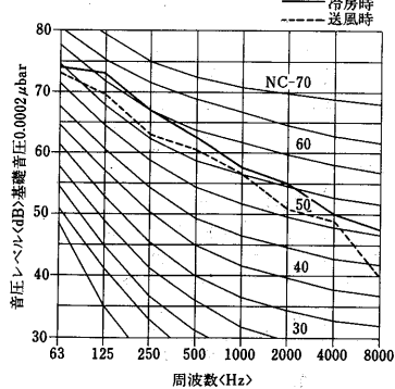
PAT-30E形 60Hz
