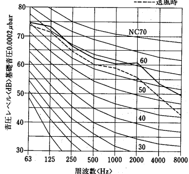
PAT-30E形 60Hz
