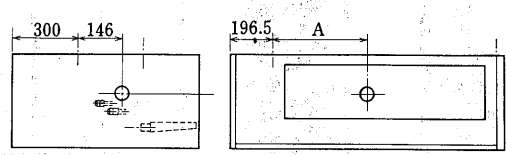
PCT-D形
