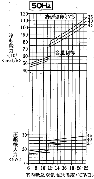
PWT-40G形 冷房能力線図
