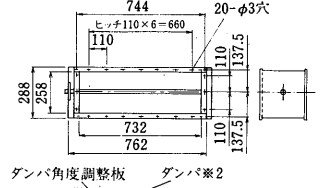
吹出ダクトフランジ詳細<別売部品> <※2ダンパ有り、ダンパ無しの2種類があります>
