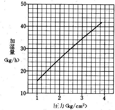
水加湿器能力線図
