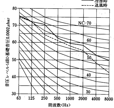
PAT-50J形
