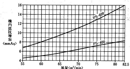
フィレドフィルタ機内抵抗線図<別売部品>
