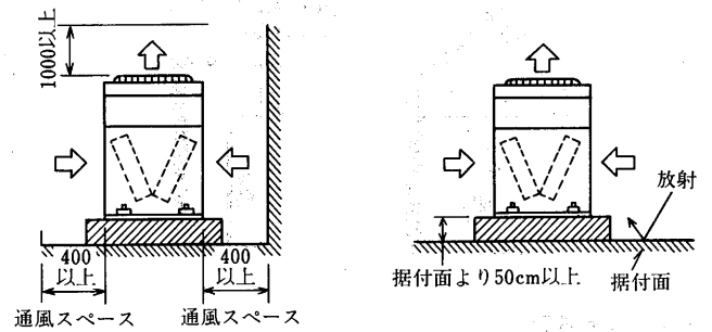
PVD-8, 10A形
