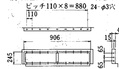
外気取入フランジ<別売部品>
