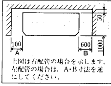
室内ユニットサービススペース
