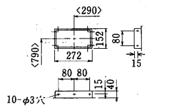
外気取入フランジ<別売部品>
