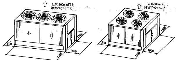
PVT-40・50J形複数台設置 PVT-40J形
