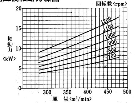
送風機軸動力線図
