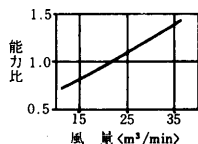
風量補正線図
