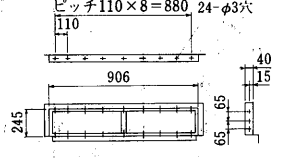
後吸込ダクトフランジ<別売部品>
