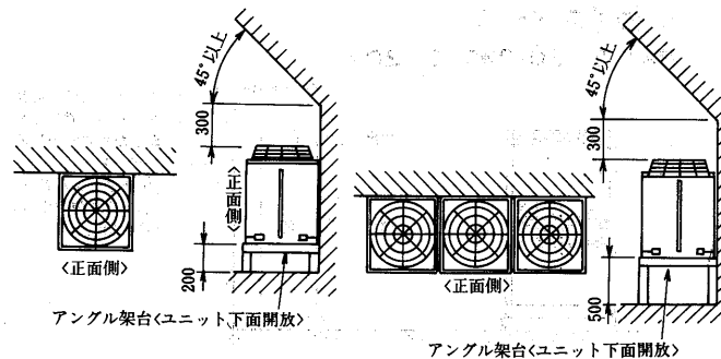
<横連続集中設置, 正面開放>
