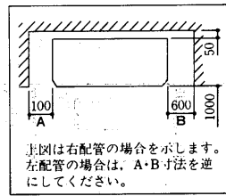
サービススペース
