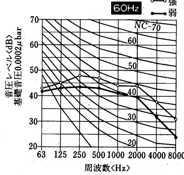
PUTF-10B形
