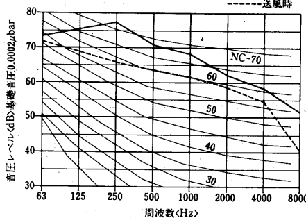
PAT-40J形
