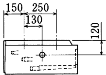
PCT-P形
