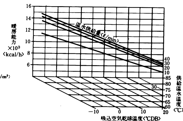
温水加熱器能力線図<2列×14段><別売部品>
