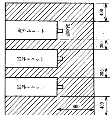
サービススペース
