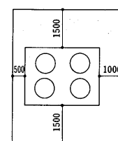
PVT-J1600J-F形 サービススペース
