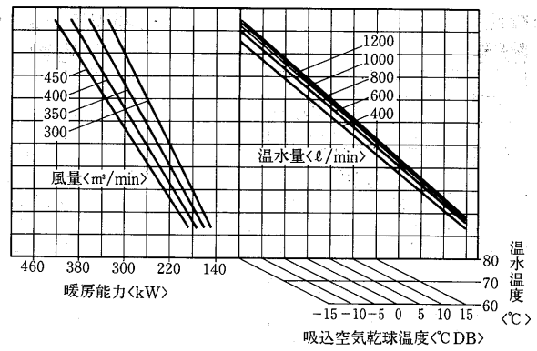
温水加熱器能力線図<2列><別売部品>
