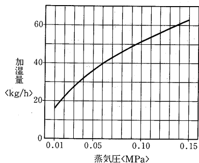
蒸気加湿器能力線図<別売部品>
