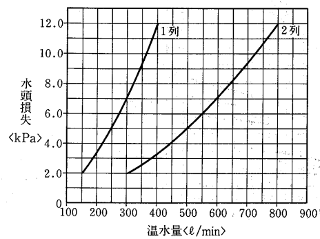
温水加熱器水頭損失線図
