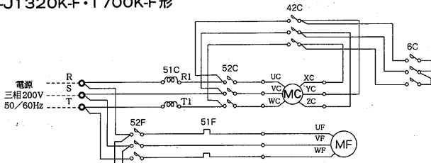
PW-J1320K-F・1700K-F形
