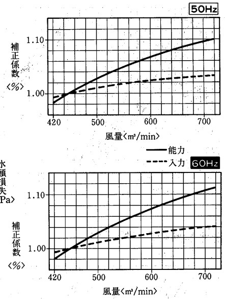
風量補正線図
