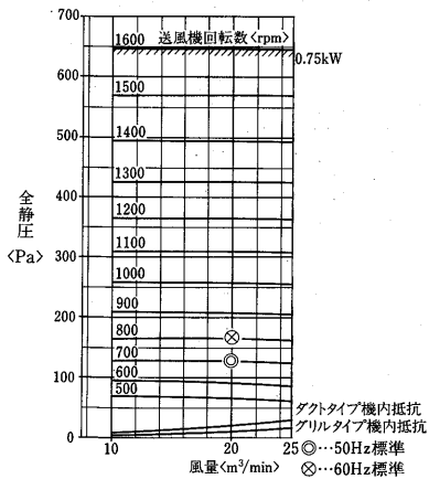
送風機性能線図
