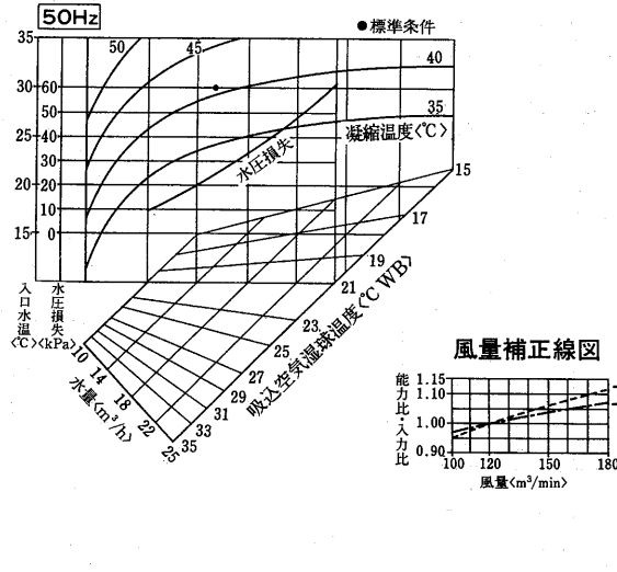
凝縮器特性線図
