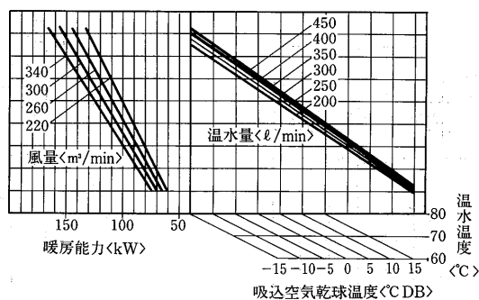
温水加熱器能力線図<1列><別売部品>
