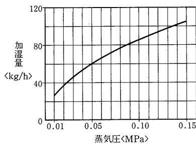
蒸気加湿器能力線図<別売部品>
