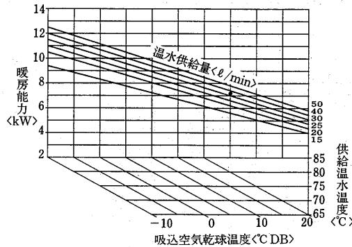
温水加熱器能力線図<別売部品>
