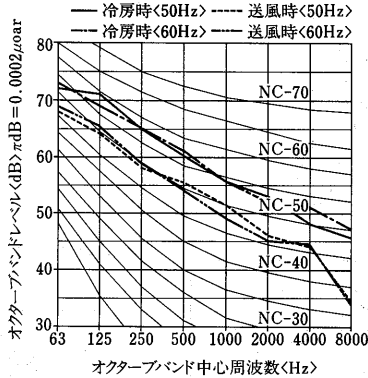
PAT-J670E-F形 PWT-J850E-F形
