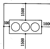
PVT-J1320J-F形 サービススペース
