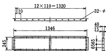
後吸込ダクトフランジ 〈別売部品〉
