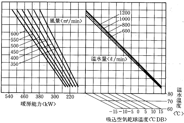
温水加熱能力線図<2列><別売部品>
