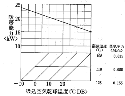
蒸気加熱器能力線図<別売部品>
