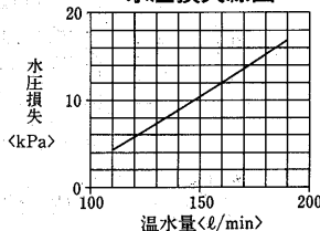
水圧損失線図
