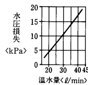
水圧損失線図
