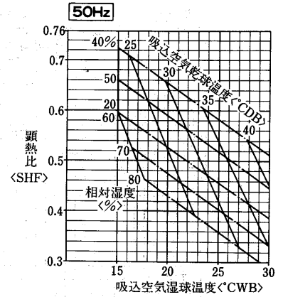
顕熱比<SHF>線図<風量20m 3 /min>
