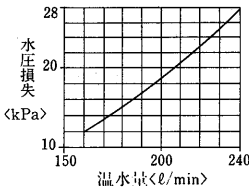
水圧損失線図
