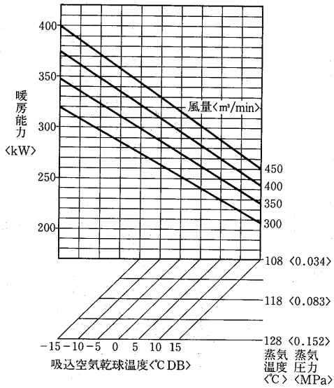
蒸気加熱器能力線図<1列><別売部品>
