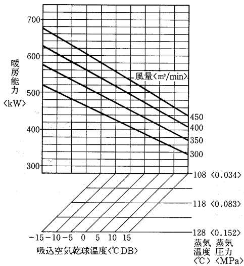
蒸気加熱器能力線図<2列><別売部品>
