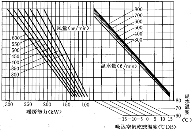
温水加熱能力線図<2列><別売部品>
