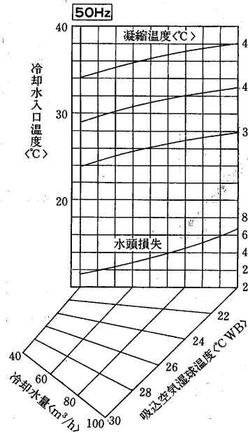
凝縮器特性線図
