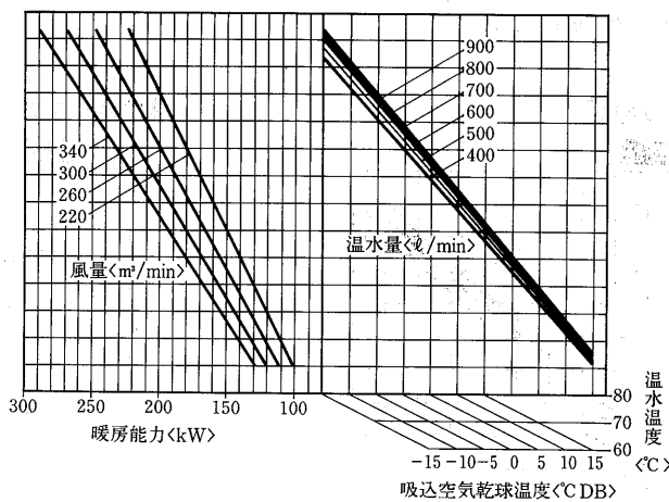
温水加熱器能力線図<2列><別売部品>
