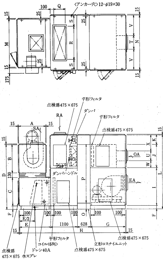
(c)排気モータ内蔵<OA100%>ゴム防振タイプ
