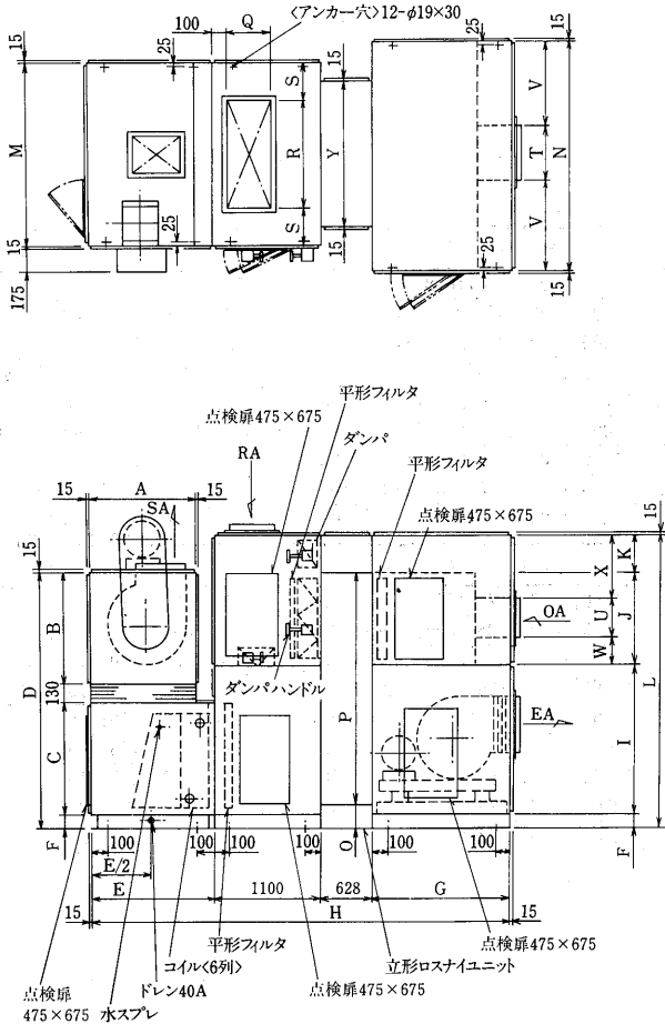
(d)排気モータ内蔵<OA30%>ゴム防振タイプ
