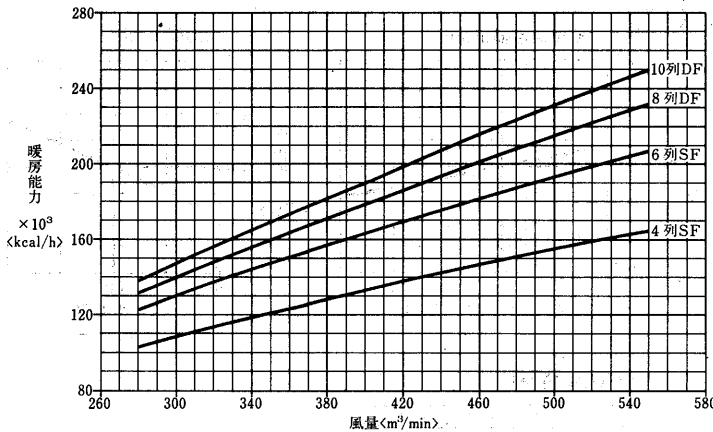
温水コイル選定図<温水60°C>
