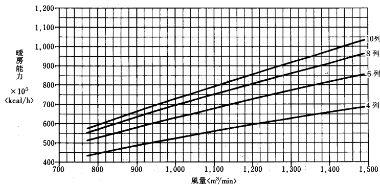
温水コイル選定図<温水60℃>
