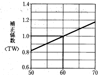
水温補正線図
