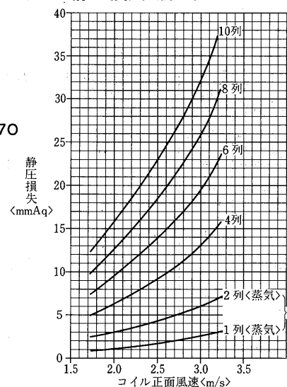
コイルの静圧損失<濡れ面>
