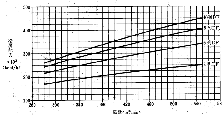
冷水コイル選定図
