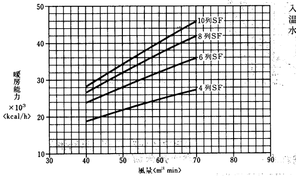
温水コイル選定図<温水60°C>
