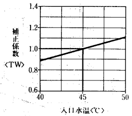
水温補正線図
