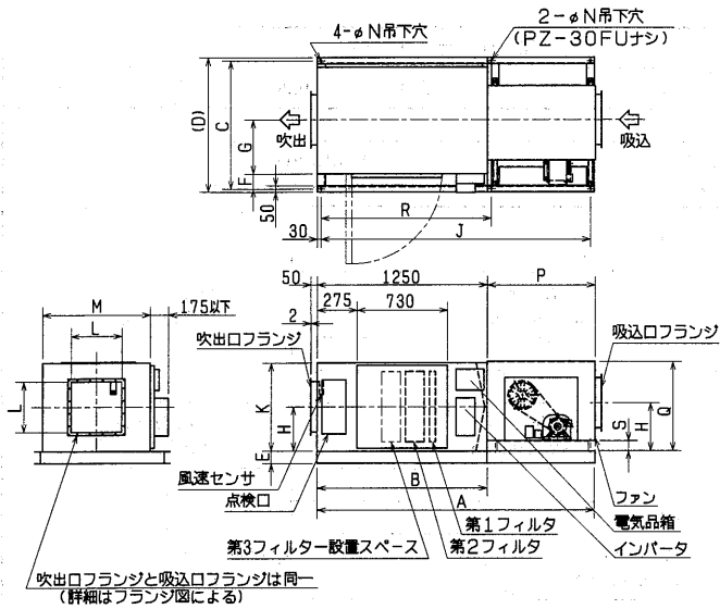
変化寸法表
