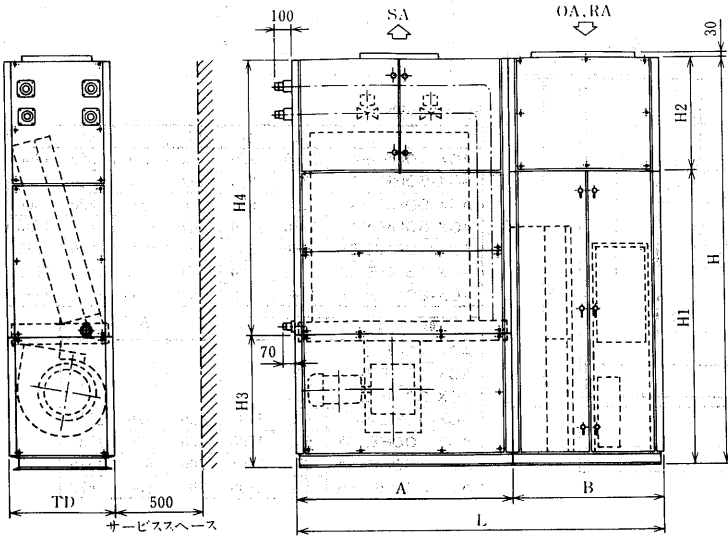
変化寸法表
