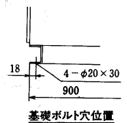
基礎ボルト穴位置
