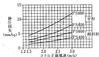
エリミネータ、縦形静圧損失線図
