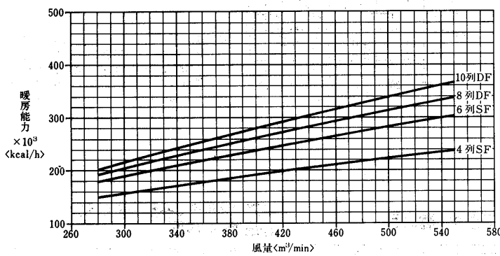
温水コイル選定図<温水60°C>
