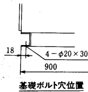
基礎ボルト穴位置
