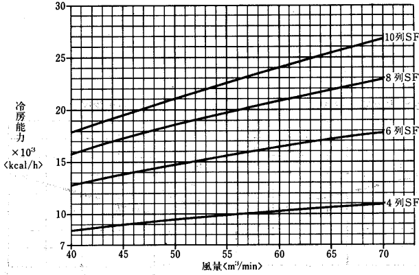
冷水コイル選定図
