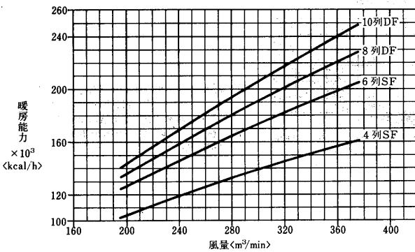
温水コイル選定図<温水60°C>
