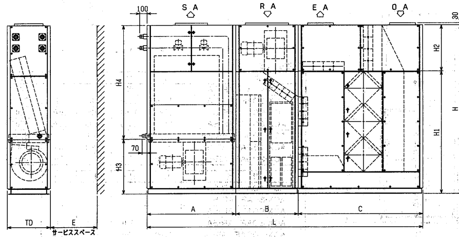
変化寸法表
