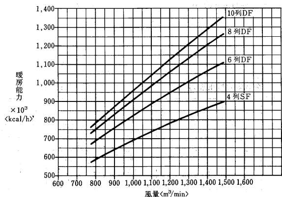
温水コイル選定図<温水60℃>
