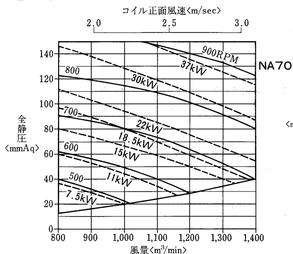
送風機能力線図
