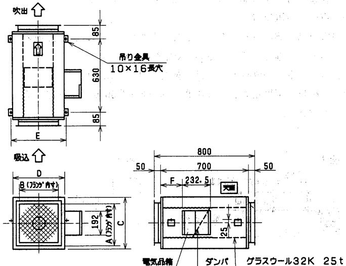
変化寸法表
