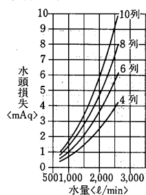
水頭損失線図
