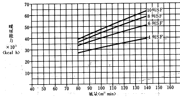
温水コイル選定図<温水45°C>
