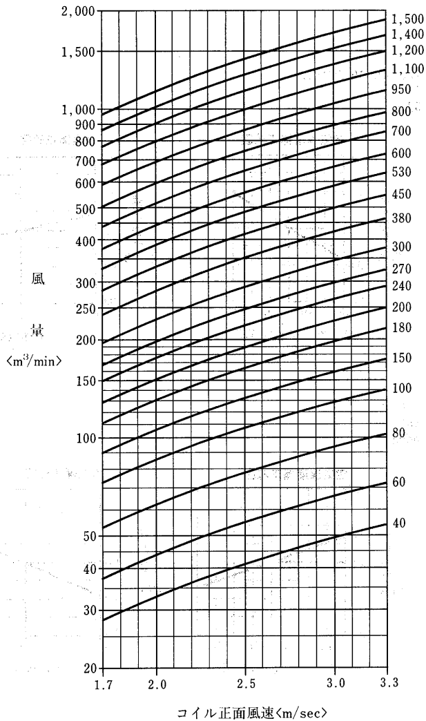
(d)ユニット形番選定線図
