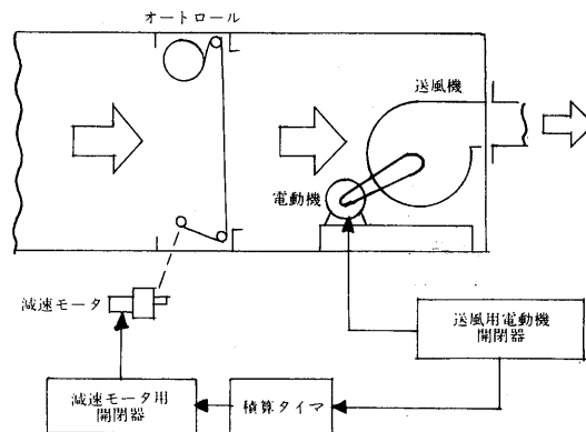
タイマ制御式の機構
