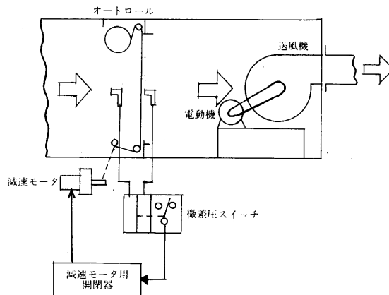
差圧制御式の機構
