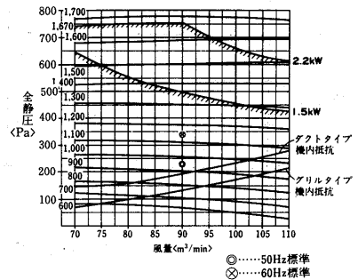
PWT-J280E-H形送風機性能線図
