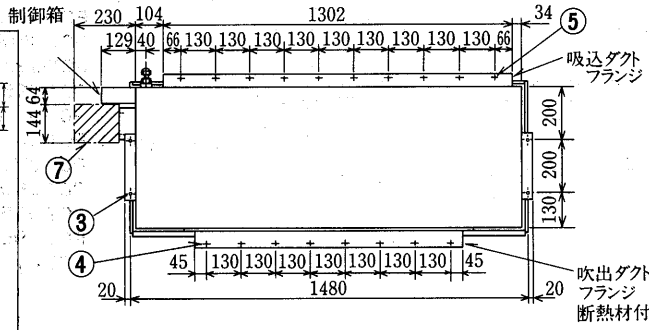
PET-J190DA形 サービススペース
