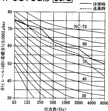
PAT-J1180J形
