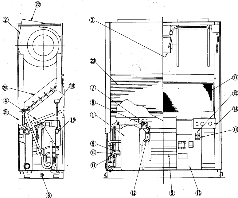
PWT-J212E形
