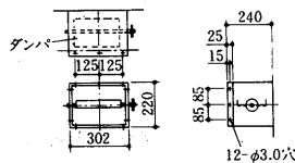
吹出ダクトフランジ<別売部品>
