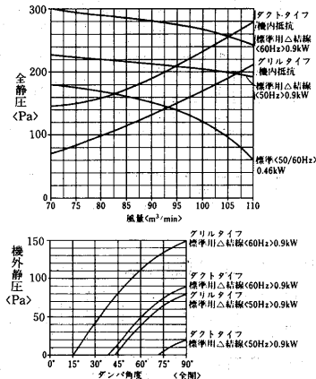
PWT-J280E形送風機性能線図
