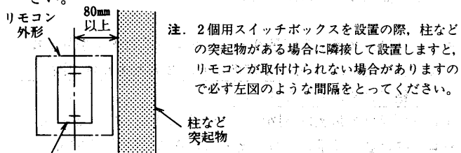
スイッチボックス
