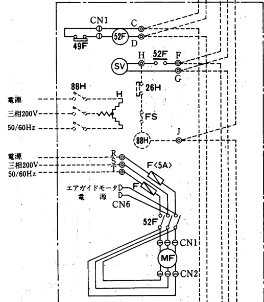
室内ユニット (PCT-J95DA・J125DA)
