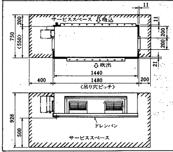
PET-J190DA形 サービススペース
