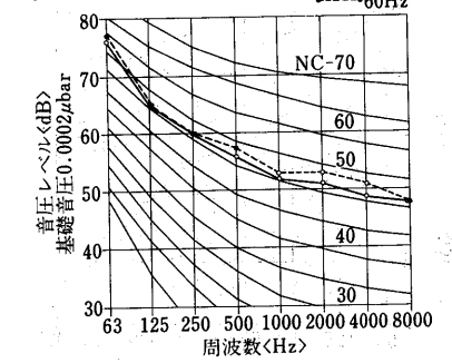
PUTS-J265B形
