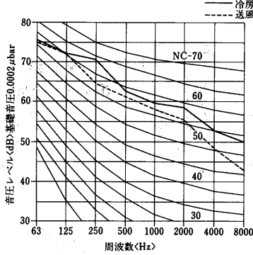
PWT-J800E形 50Hz
