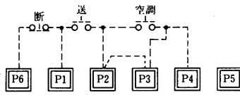
⑪DC24Vトグルスイッチ方式
