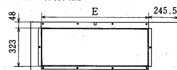
本体取付背面図
