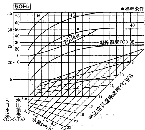
PWT-J280E<H>形 凝縮器特性線図
