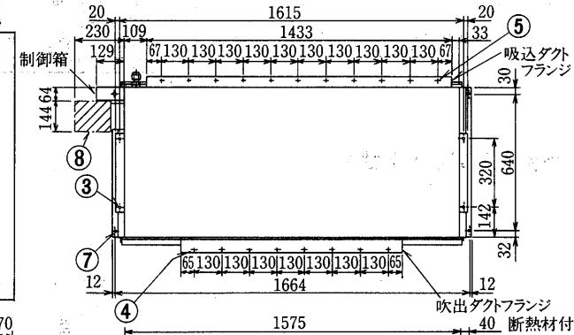
PET-J250DA形 サービススペース
