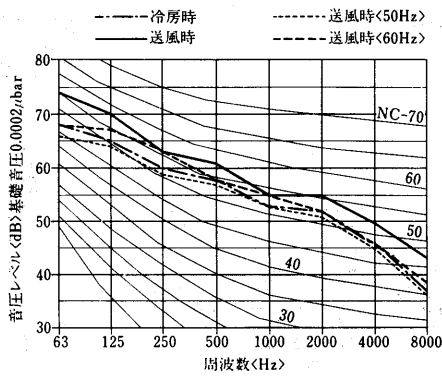
PWT-J560E形
