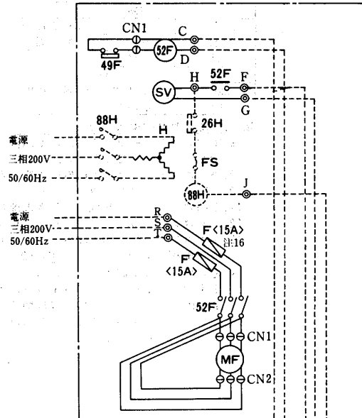
室内ユニット <PET-J190DA・J250DA・J375DA>
