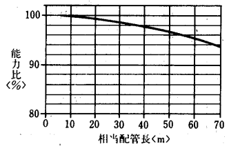
PAT-J530G形
