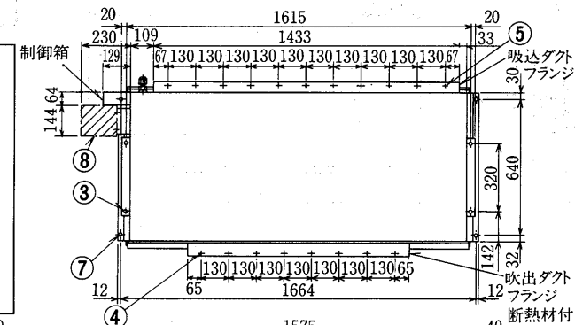
PET-J375DA形 サービススペース
