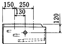
PCT-P形
