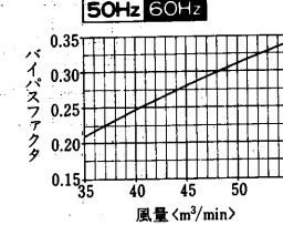
バイパスファクタ線図 50Hz 60Hz
