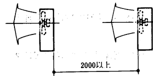
室外吹出ガイド不使用<冷房に限る>
