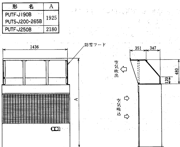
防雪フード<F-75C形>
