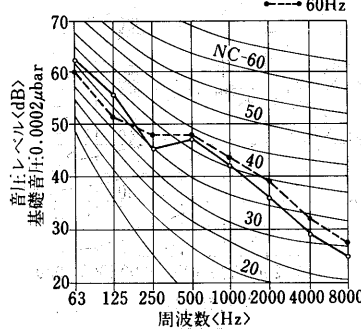
PUTS-J200B形
