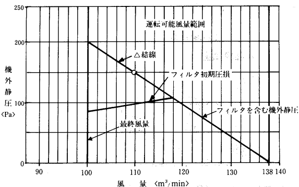
PET-J250DA形
