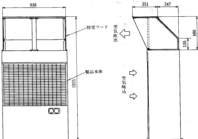
防雪フード<F-45C形>
