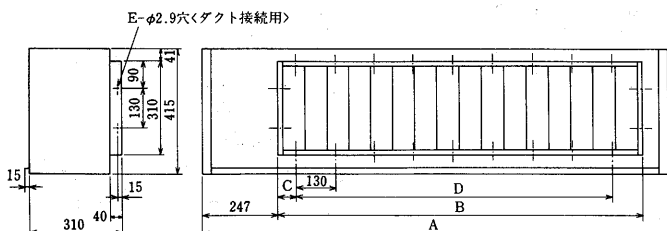
変化寸法表
