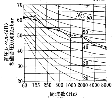
PUT-J50A形
