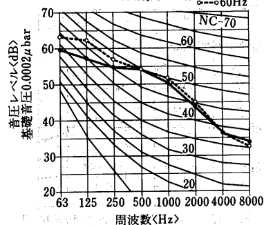
PUTS-J118B形
