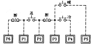
⑥トグルスイッチ方式 冷暖切換方式
