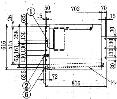
PET-J375DA形 サービススペース
