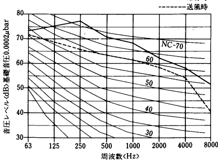
PWT-J1000G形
