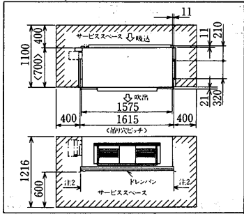
PET-J250DA形 サービススペース
