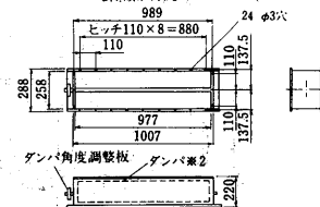
吹出ダクトフランジ<別売部品> (※2ダクト有り、ダンパ無し 2種類があります)
