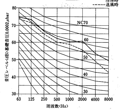
PWT-J800E形 60Hz
