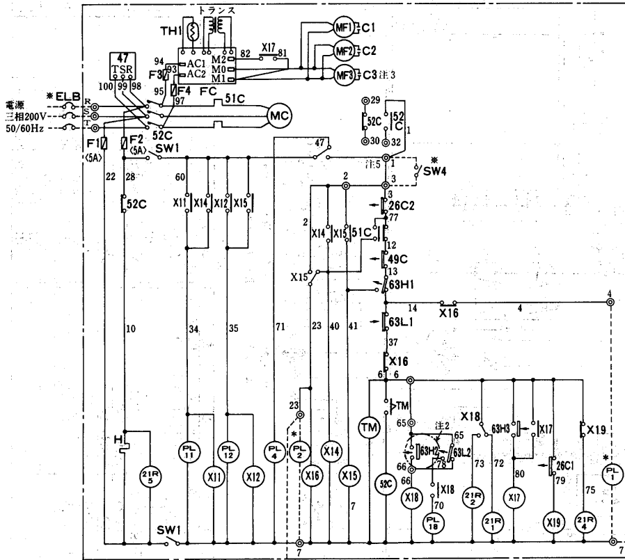
室外ユニット(PUTF-J125・190・250B)
