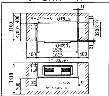
PET-J375DA形 サービススペース
