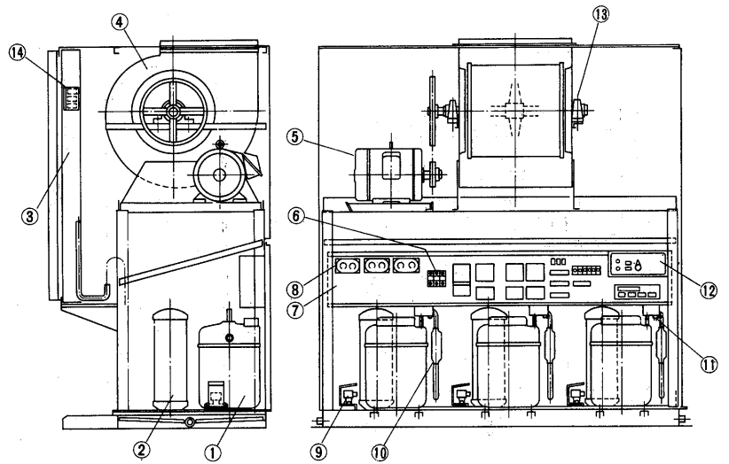
PAT-J530G形<室内ユニット> PAT-J670G形
