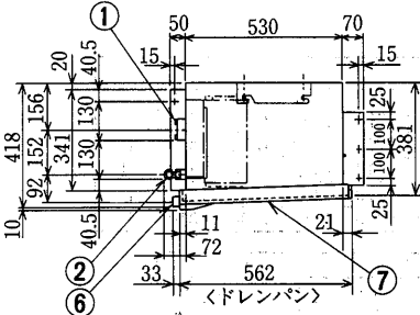
PET-J250DA形 サービススペース
