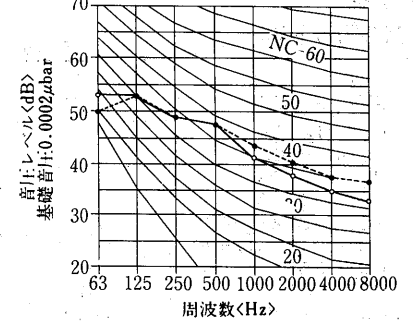
PUTF-J125B形
