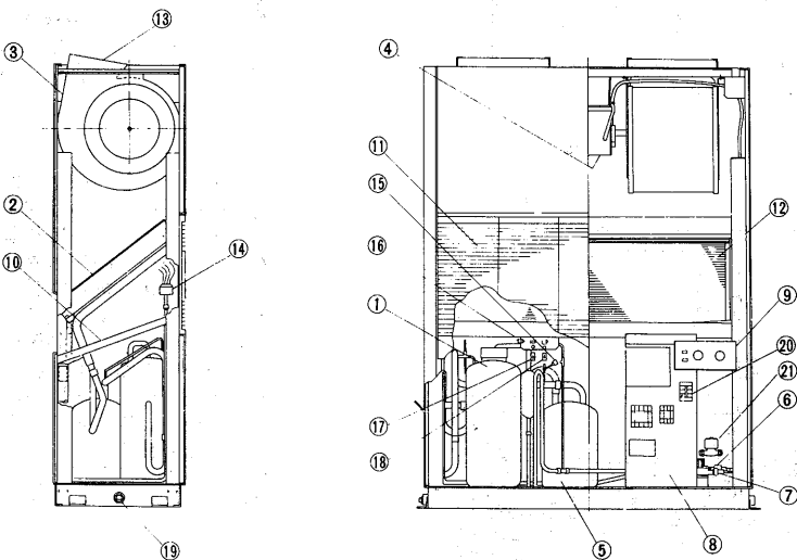
PAT-J190G形<室内ユニット>
