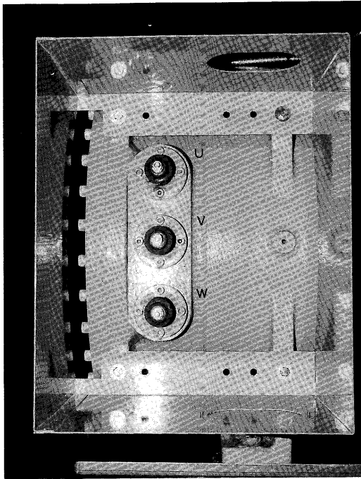
図3. モータ端子
