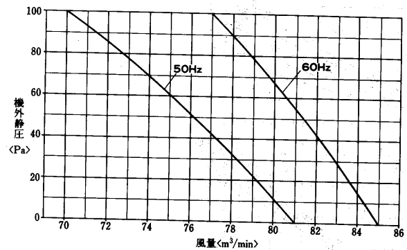
KFH-5NA1形
