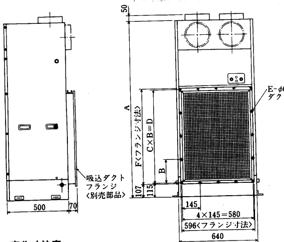
変化寸法表
