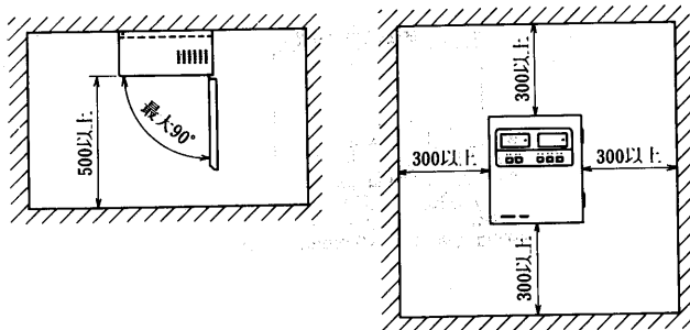
サービススペース
