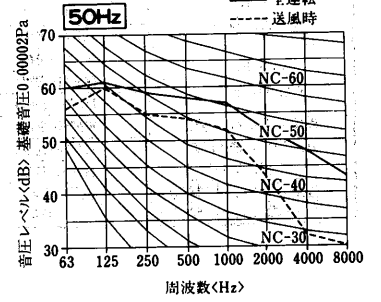
RFH-5B 1 形
