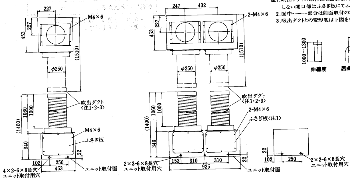
J-3NFD形
