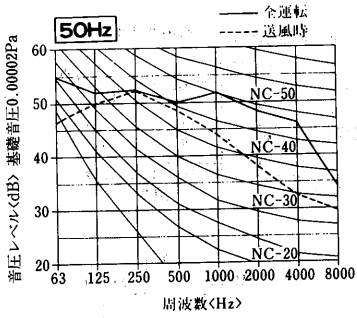
RFH-2B 1 形
