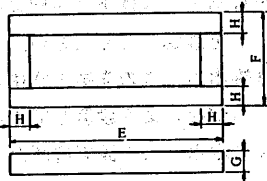
据付台寸法図(別売部品) PAC-CQ33MD
