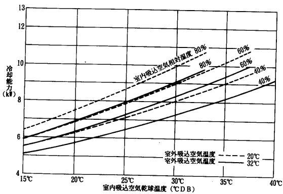
RFH-3B 1 形 50Hz
