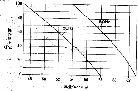
RFH-5B 1 形
