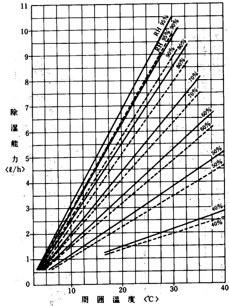
RFH-3B1形
