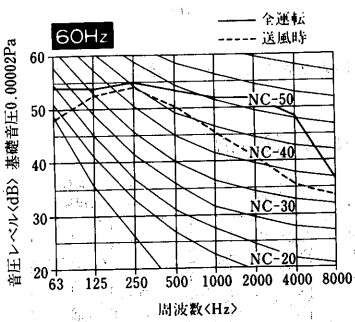
RFH-2B 1 形
