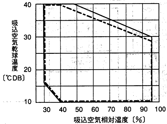
RFH-10A形
