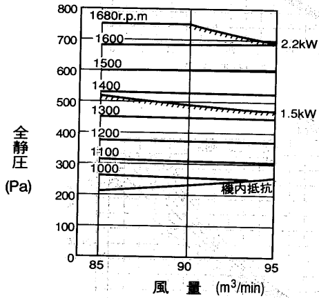
RFH-10A形
