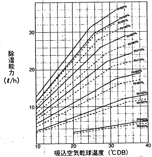
RFH-10A形
