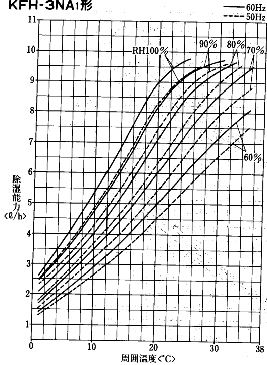
KFH-3NA1形
