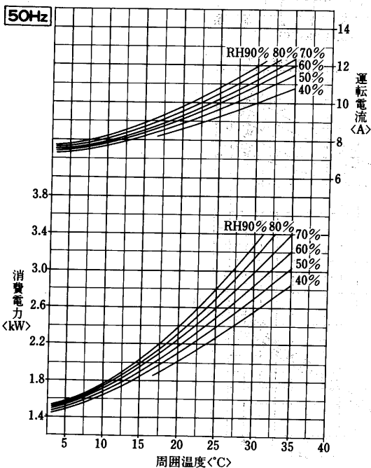
KFH-3NA1形
