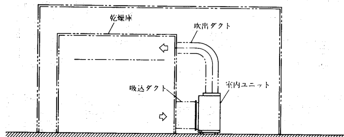
据付要領
