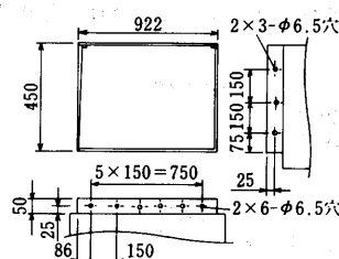
吹出口ダクト接続部詳細
