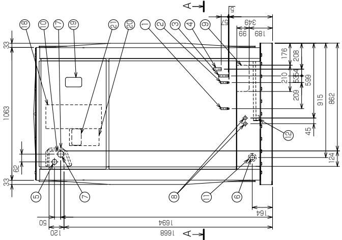
左側面図
