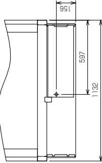
断面A-A
