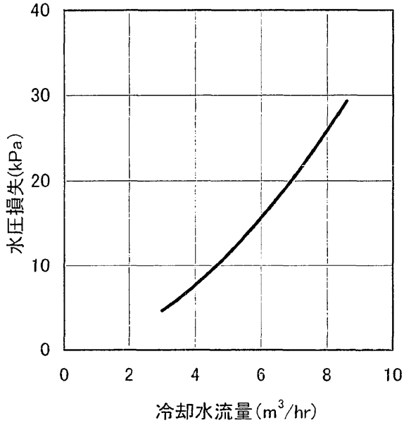
冷却器水圧損失
