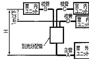
〈冷媒配管工事制限〉
