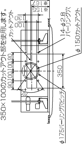
分ダクト接続口詳細図(両側面)
