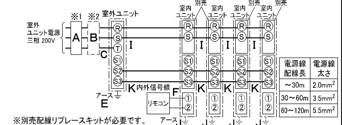
(3) 室 外 ユ ニ ッ ト 以 上 室 内 ユ ニ ッ ト に 電 源 を 供 給 す る 方 式
