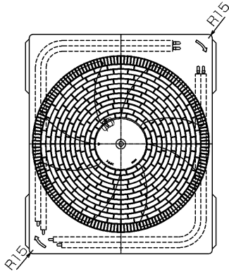
右側面図
