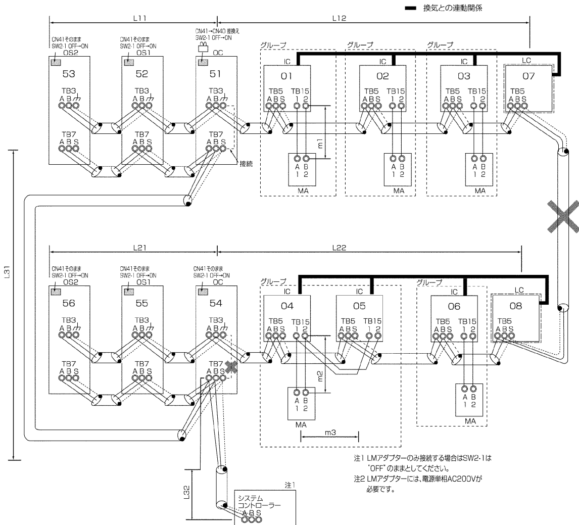
制御線配線例
