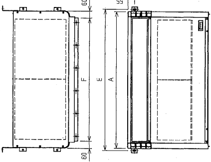
別売吹出ダクトフランジ組込時
