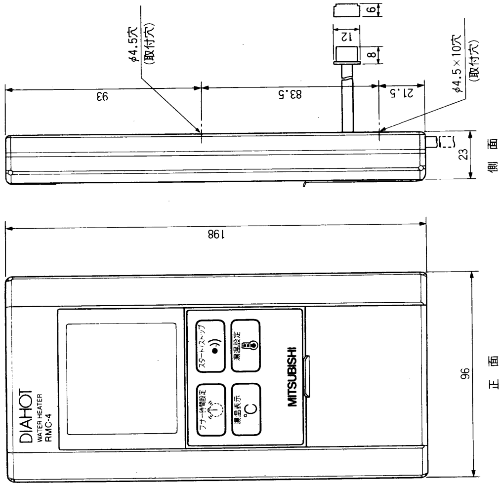
リモコン外形寸法図(RMC-4)
