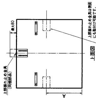
脚固定金具使用時(上面透視図)
