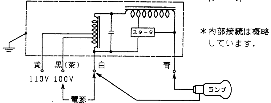
結線図
