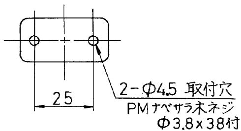
引掛シーリング取付寸法図
