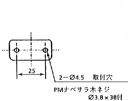
引掛シーリング取付寸法図
