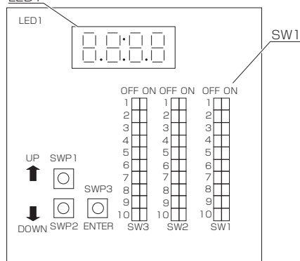
LED1 マイコン基板上ディップスイッチ
