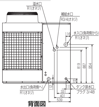
MCAV-P300A-PT形
