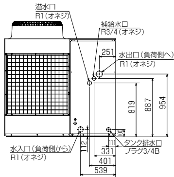
背面図
