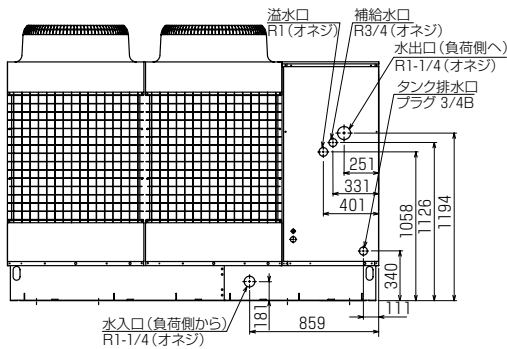
背面図
