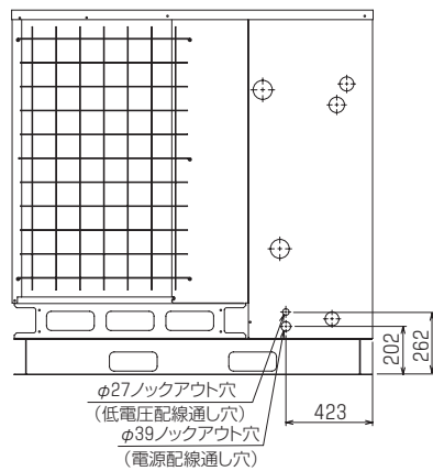
背面図
