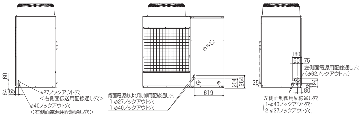
右側面図
