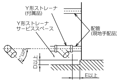
取付例2
