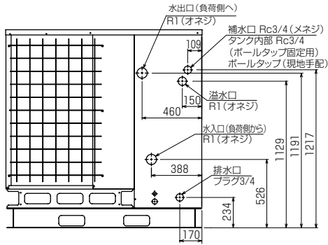
背面図
