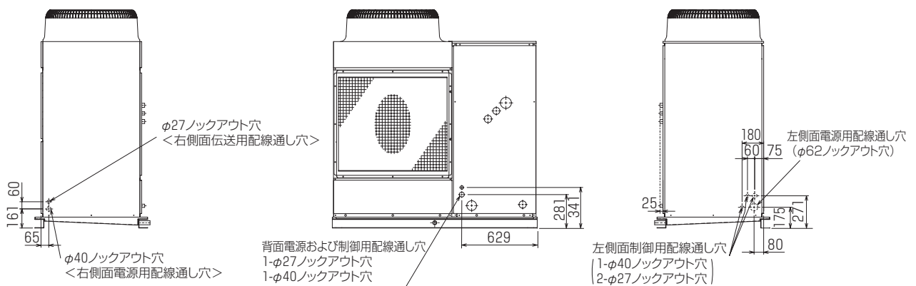
右側面図
