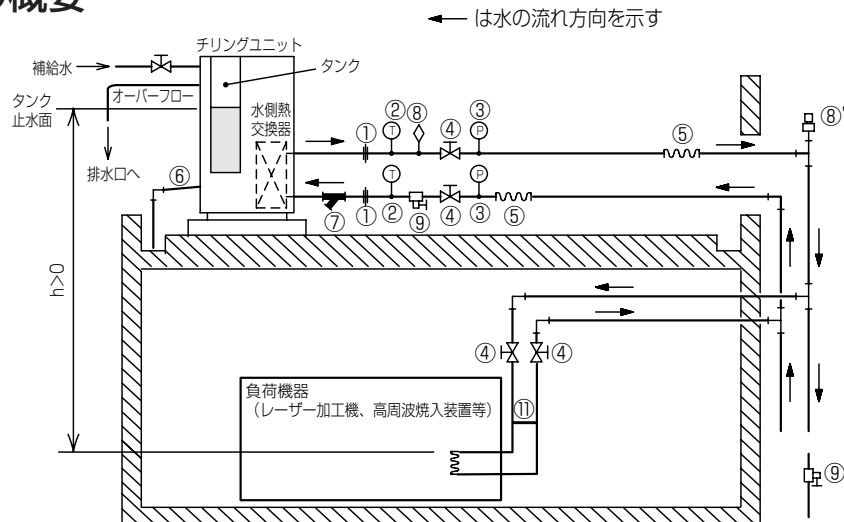
図4-1 水配管構成図
