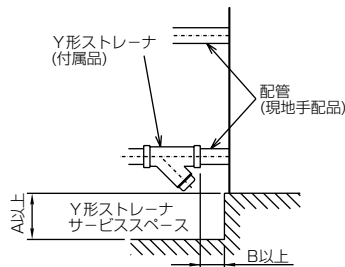
取付例1
