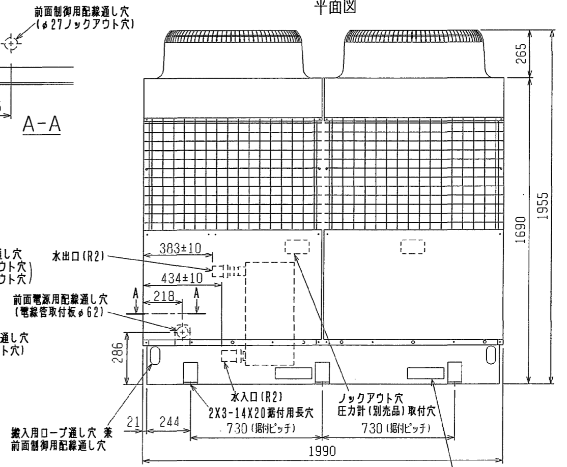
正面図
