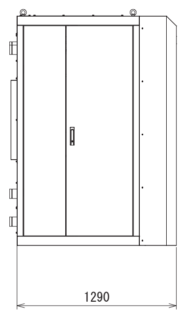
<左側面>
