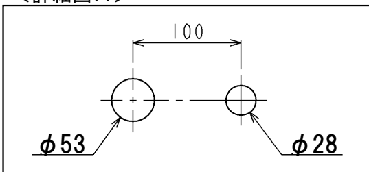
<詳細図 A>
