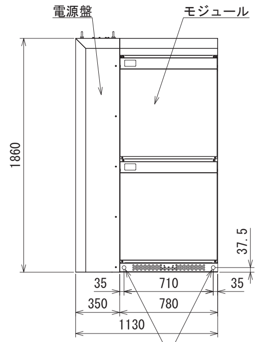
<サビス面> (反サビス面側共) 吊位置
