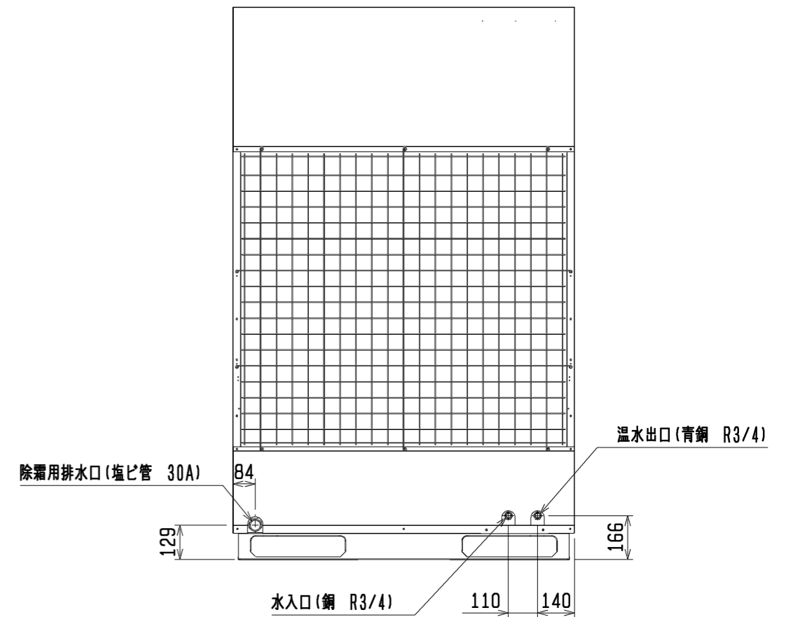
背面図
